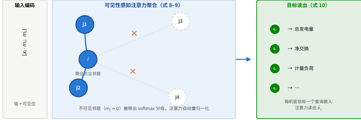
图 2 可见性感知的图消息传递与目标读出。节点输入同时编码字段值和可见位；不可见邻居被移出注意力归一化，每个机密目标再由独立查询向量读取相应的字段子图表示。
