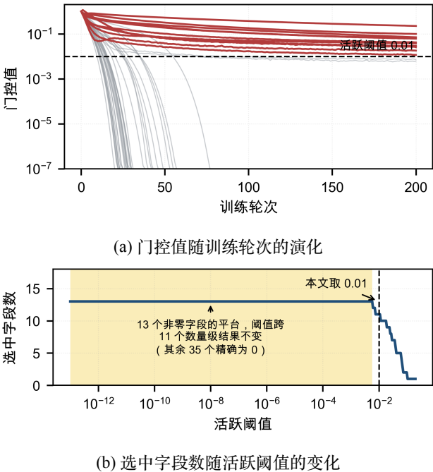
图 3 净实际交换功率的门控值演化与阈值敏感性 Fig. 3 Gate evolution and threshold sensitivity for net actual interchange
