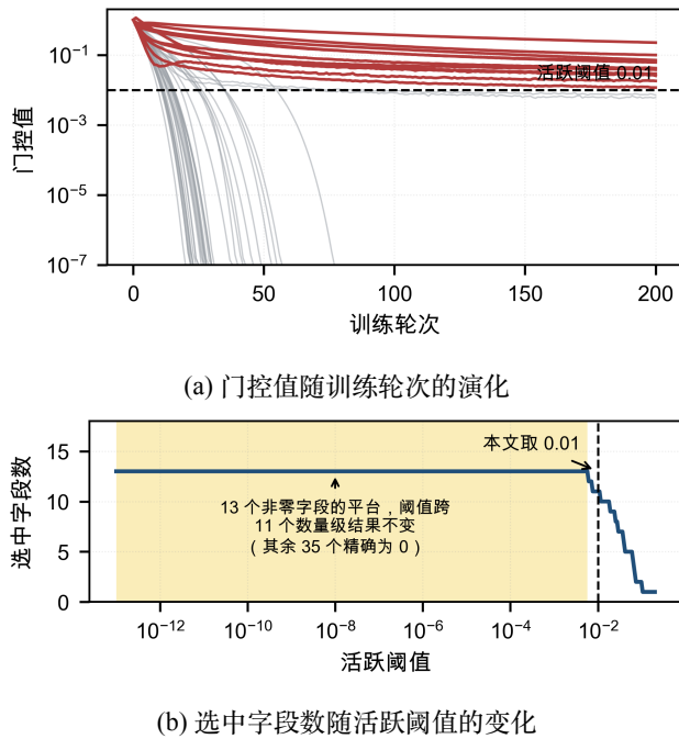
图 2 净实际交换功率的门控值演化与阈值敏感性 Fig. 2 Gate evolution and threshold sensitivity for net actual interchange
