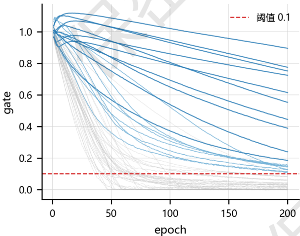
图 6 净实际交换功率目标上门控参数的演化过程 Fig. 6 Evolution of gate parameters for net actual interchange
