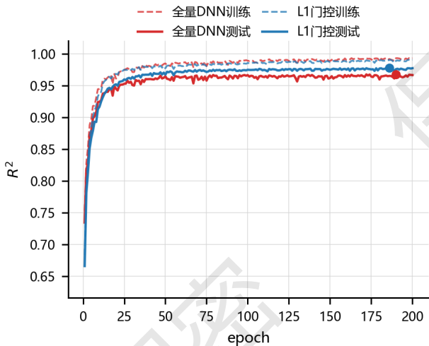
图 5 净实际交换功率目标上的 R^2 训练过程对比 Fig. 5 Comparison of training R^2 processes for net actual interchange
