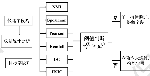
图 2 多相关性初筛流程
