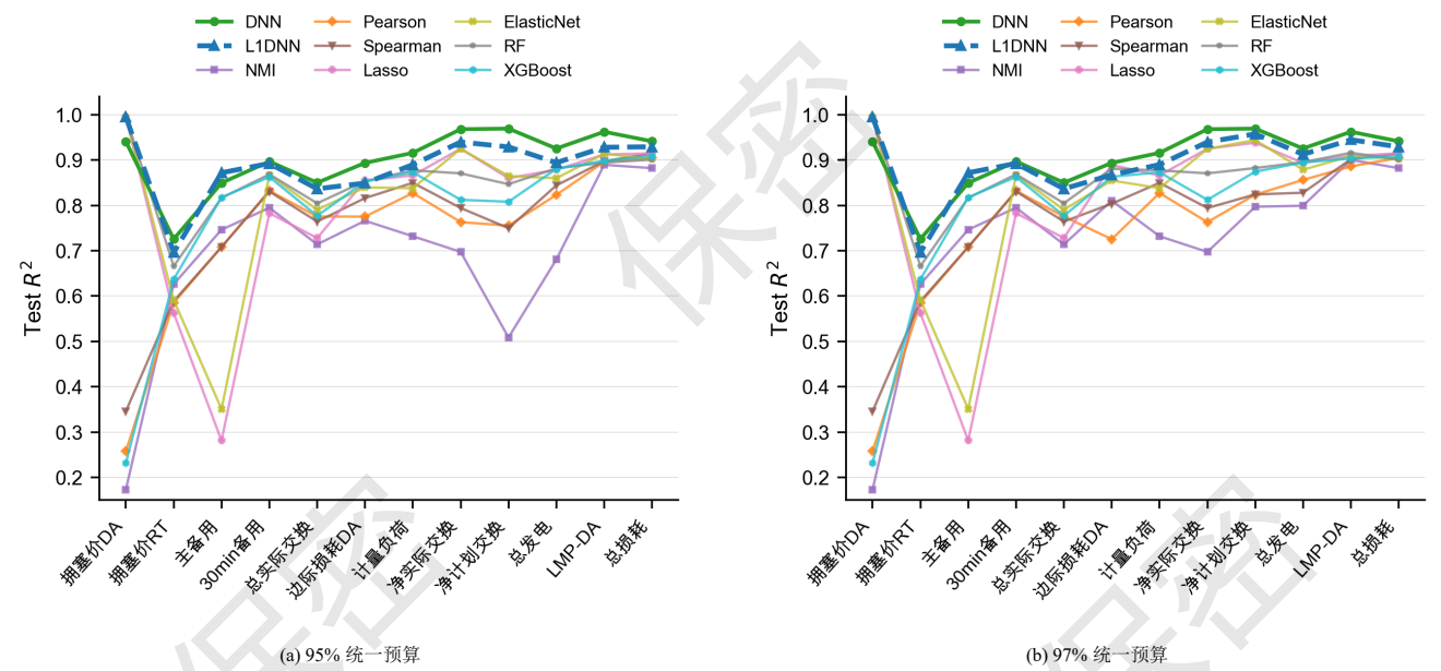
图 10 统一预算下 9 种方法的目标级测试 R^2 对比 Fig. 10 Target-level comparison of 9 methods under unified feature budgets
