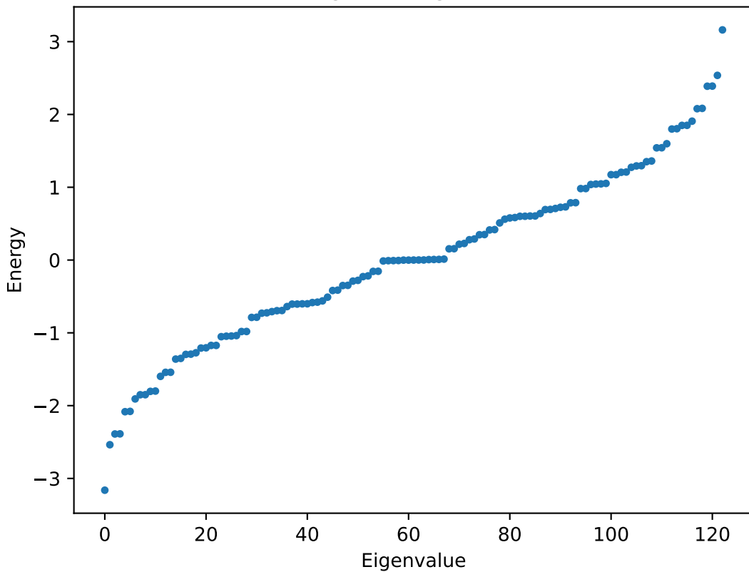
Energies of Eigenvalues
