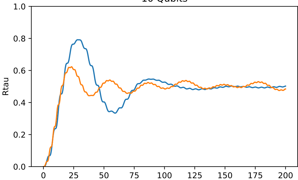
10 Qubits
