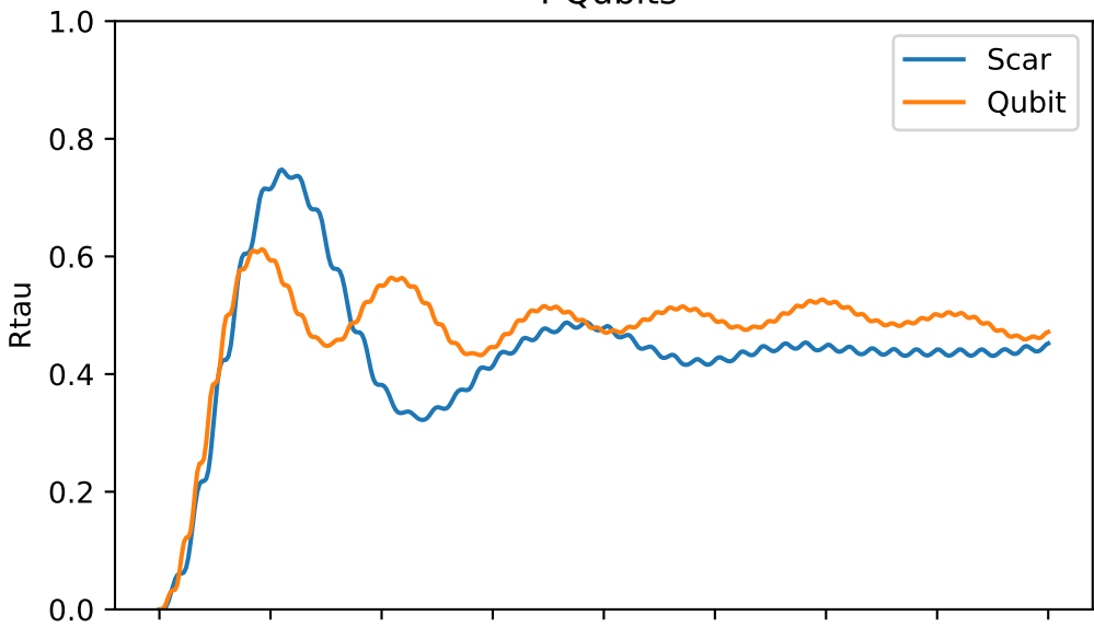
4 Qubits
