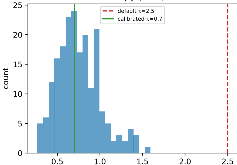
Entropy (nats)
