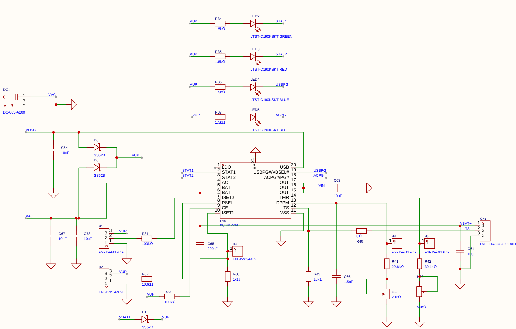
USB-电池供电切换电路
