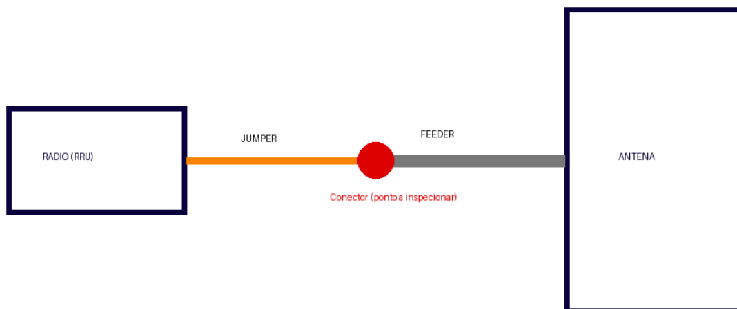
Figura 1 — Ligação rádio, jumper, feeder e antena.
