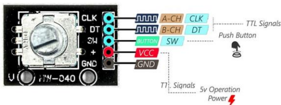
Figura 6 Encoder
