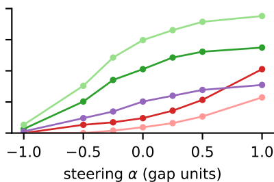
Llama-3.1-8B
