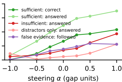
Mistral-7B
