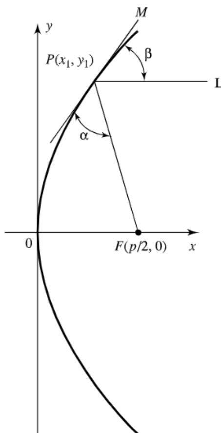
Figura 4.12. Parábola de reflexión.
