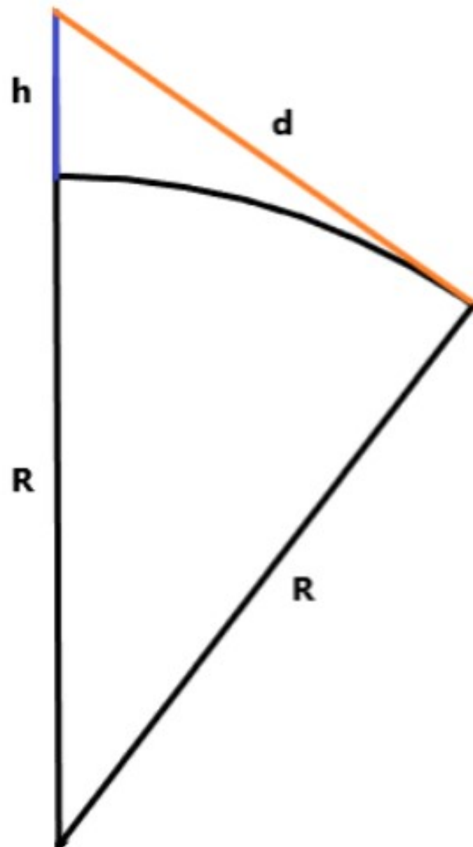
Figura 1. Geometría de la línea de visión
