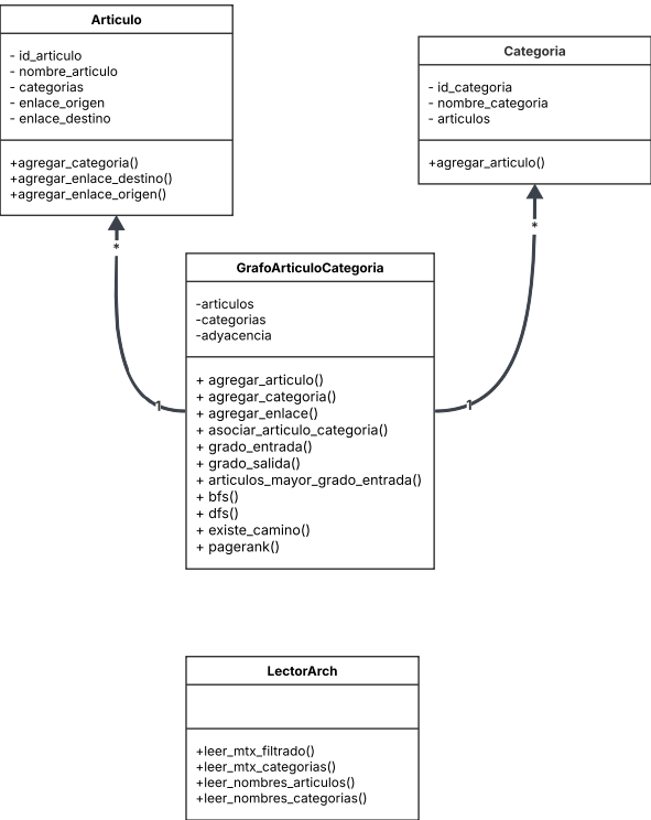
Figura 1. Diagrama de clases del sistema implementado. Fuente: elaboración propia.
