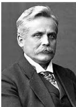
6. ábra. Balra: Wilhelm Wien (1864–1928). Jobbra: az AFT sugárzásának spektrális eloszlása néhány hőmérsékleten. Ahogy a hőmérséklet nő, a görbe magasabb, maximuma ( \lambda_{\max} ) pedig a rövidebb hullámhosszak felé tolódik (szaggatott vonal).
