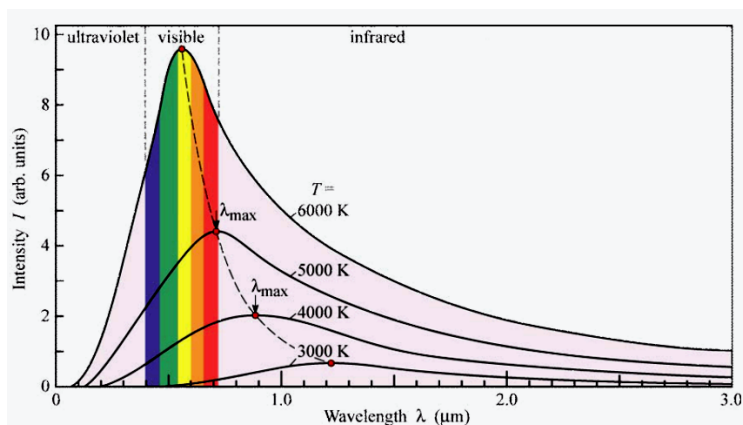
6. ábra. Balra: Wilhelm Wien (1864–1928). Jobbra: az AFT sugárzásának spektrális eloszlása néhány hőmérsékleten. Ahogy a hőmérséklet nő, a görbe magasabb, maximuma ( \lambda_{\max} ) pedig a rövidebb hullámhosszak felé tolódik (szaggatott vonal).
