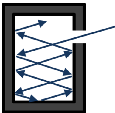
4. ábra. Az abszolút fekete test modellje. A kis nyíláson belépő sugár annyiszor verődik vissza a belső falakról, hogy azok teljesen elnyelik. Ezért látszik a nyílás tökéletesen feketének.
