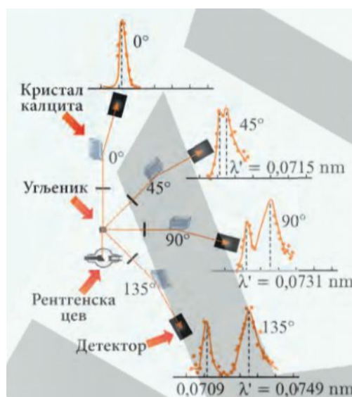
Слика 13. Шема Комптоновог експеримента. Рендгенско зрачење пада на угљеник (графит), расејава се под различитим угловима, а измерена таласна дужина расте са углом расејања (нпр. 0,0709 \text{ nm} на 0^\circ , 0,0731 \text{ nm} на 90^\circ , 0,0749 \text{ nm} на 135^\circ ).
