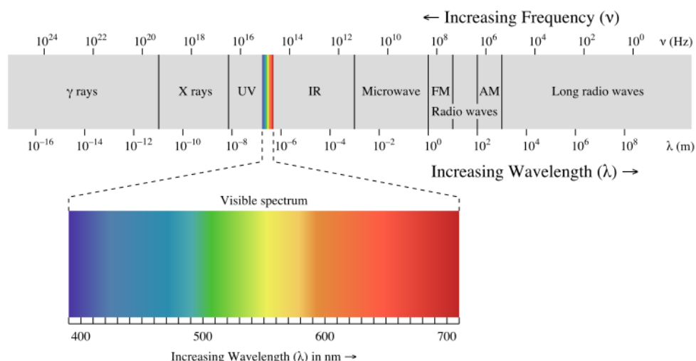
Слика 2. Спектар електромагнетног зрачења. Видљива светлост је само уска трака између инфрацрвеног (топотног) и ултраљубичастог дела. Топотно зрачење тела на собним температурама лежи у инфрацрвеном, за нас невидљивом делу.
