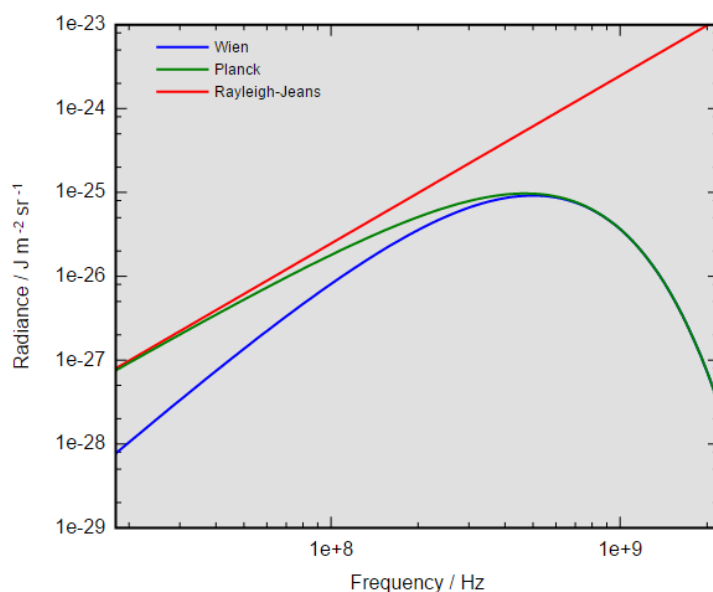
Слика 8. Поређење теорија. Класична Рејлеј--Џинсова крива (горња права која расте у недоглед) слаже се са експериментом само на малим фреквенцијама, а затим бежи ка бесконачности — ултраљубичаста катастрофа. Планкова крива прати експеримент на свим фреквенцијама.
