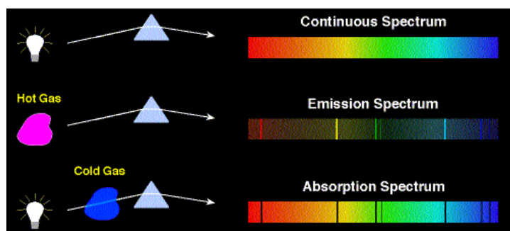
Слика 3. Три врсте спектра. Усијано чврсто тело даје континуалан спектар (све боје). Врели гас даје емисиони линијски спектар (светле линије), а хладан гас испред извора апсорбује исте те линије (апсорпциони спектар).
