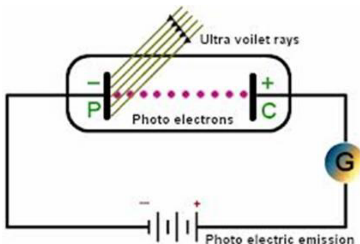
Слика 10. Шема апаратуре за фотоефекат. Светлост (у примеру ултраљубичаста) пада на катоду, из ње избија електрон (фотоелектрон) који путује ка аноди; галванометар G мери насталу струју.
