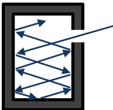
Слика 4. Модел апсолутно црног тела. Зрак који уђе кроз отворчић толико пута се одбије о унутрашње зидове да га они у потпуности апсорбују. Зато отвор изгледа савршено црно.
