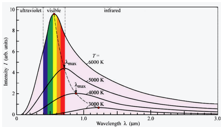
Слика 6. Лево: Вилхелм Вин (1864–1928). Десно: спектрална расподела зрачења АЦТ на неколико температура. Како температура расте, крива је виша, а њен максимум ( \lambda_{\max} ) помера се ка краћим таласним дужинама (испрекидана линија).
