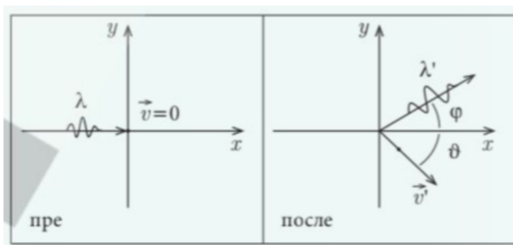
Слика 14. Судар фотона и електрона (лево „пре”, десно „после”). Пре судара електрон мирује ( \vec{v} = 0 ), а фотон има таласну дужину \lambda . После судара фотон има већу таласну дужину \lambda' и одлази под углом \varphi , док електрон одлеће под углом \vartheta брзином \vec{v}' .
