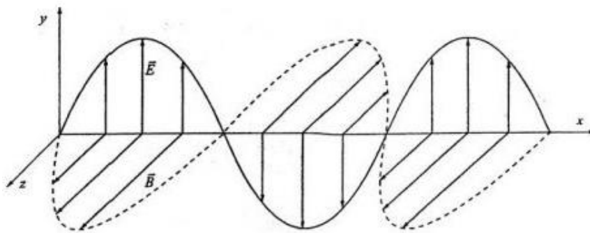
Слика 1. Електромагнетни талас: вектори електричног поља \vec{E} и магнетног поља \vec{B} узајамно су нормални и нормални на правац простирања. Зато је талас трансверзалан.
