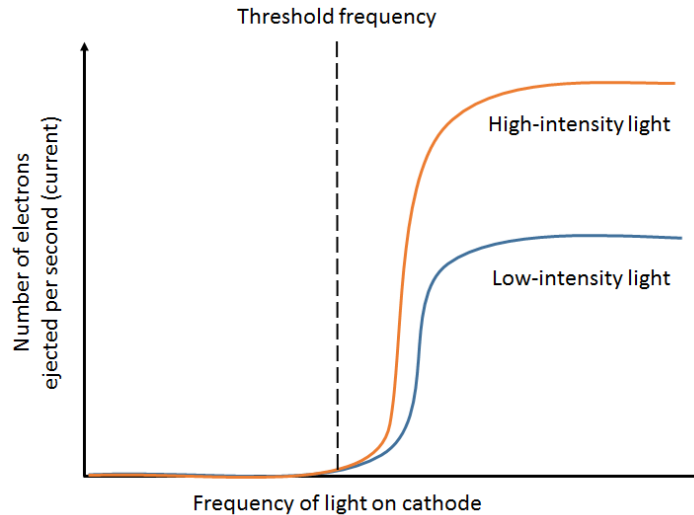
Слика 11. Зависност од фреквенције светлости. Испод граничне (прагова) фреквенције нема фотоелектрона, без обзира на интензитет. Јача светлост (горња крива) даје више електрона, али праг остаје исти.
