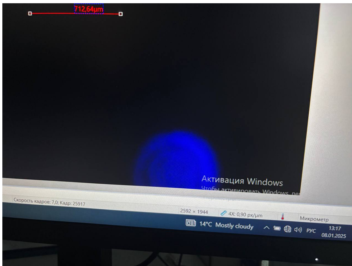
Рис. 22: Дифракция Френеля на отверстии с темными кольцами
