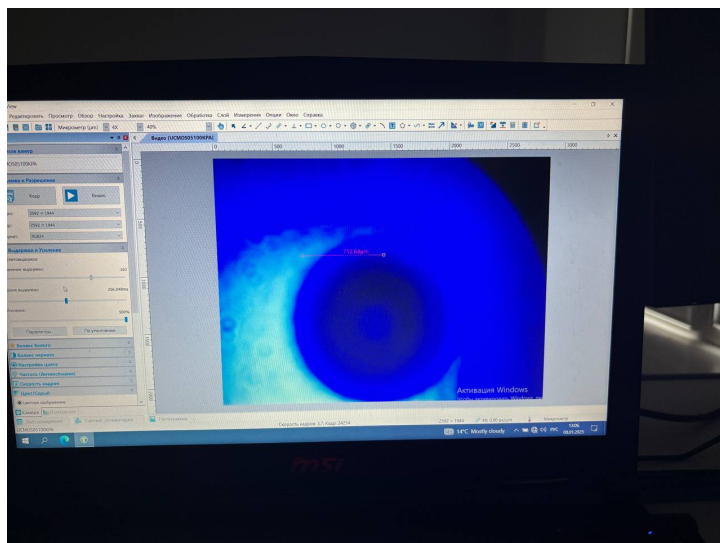
Рис. 20: Светлое пятно при другом препятствии
