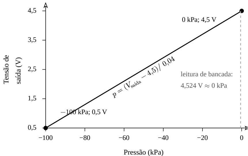
Figura 3 – Curva nominal de conversão do transdutor XGZP6847A100KPGN
