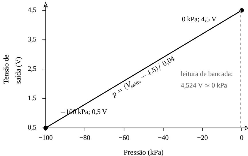
Figura 3 – Curva nominal de conversão do transdutor XGZP6847A100KPGN
