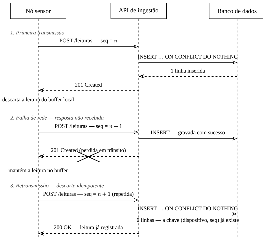
Figura 5 – Contrato de ingestão de leituras, com retransmissão e descarte idempotente
