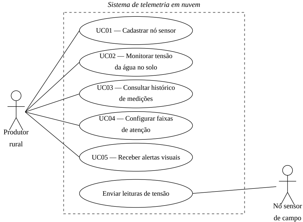
Figura 2 – Diagrama de casos de uso do sistema de telemetria
