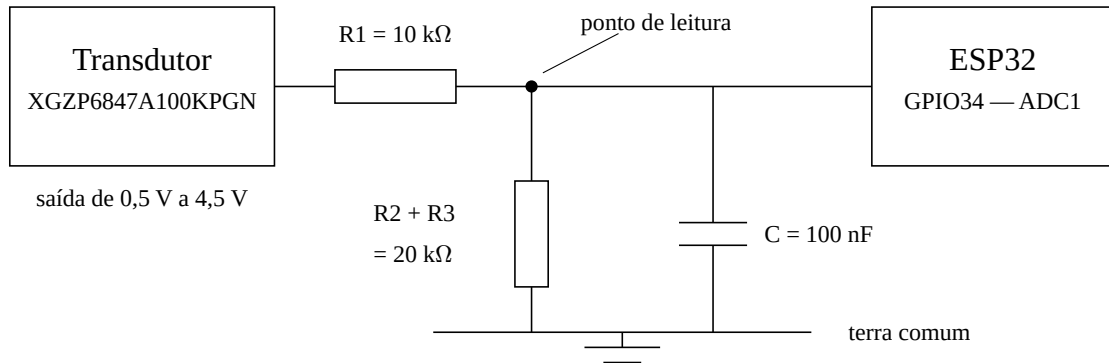
Figura 4 – Esquema do circuito de condicionamento do sinal
