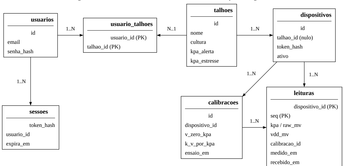
Figura 6 – Modelo de entidades e relacionamentos do serviço de retaguarda
