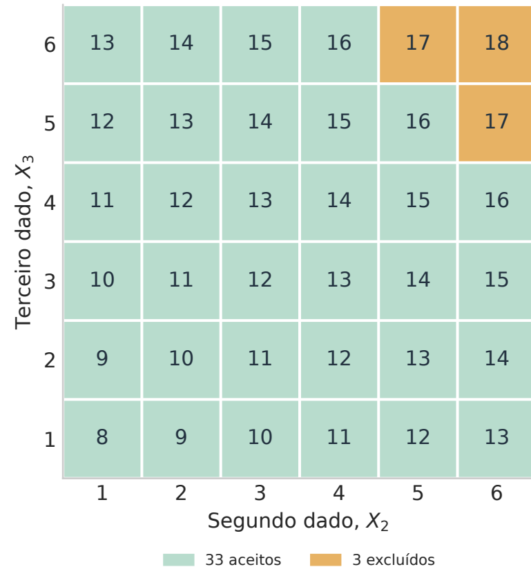
(c) Os 36 resultados com X_1 = 6
