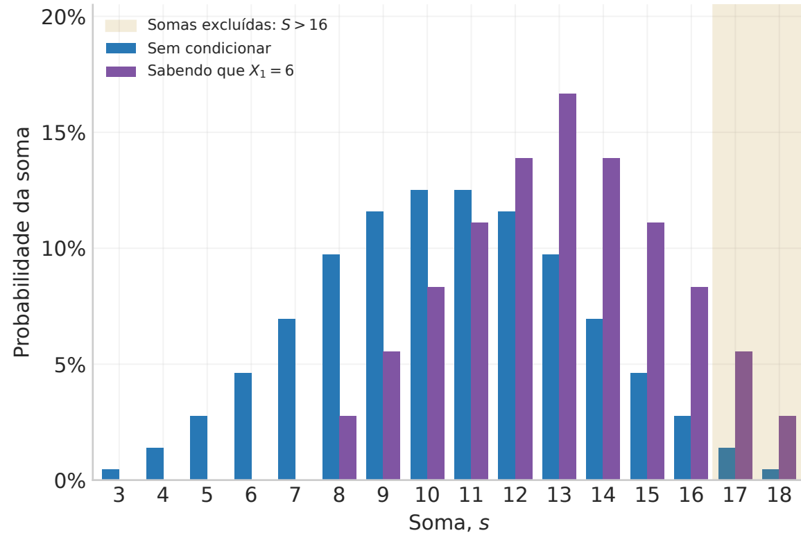
(b) e (c) A informação muda a distribuição
