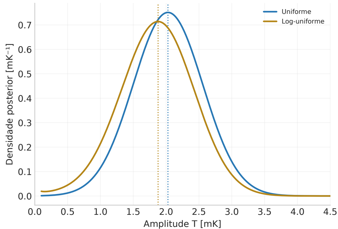
(d) Posterior de T: M1 e centro 24 assumidos
