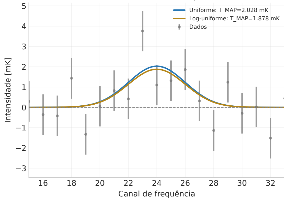
Perfis físicos nas modas das posteriores
