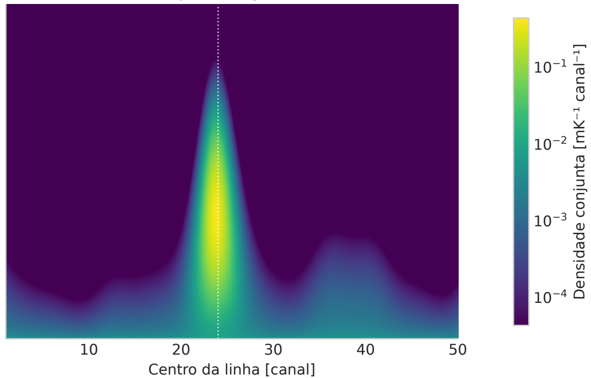
(f) Conjunta: Log-uniforme
