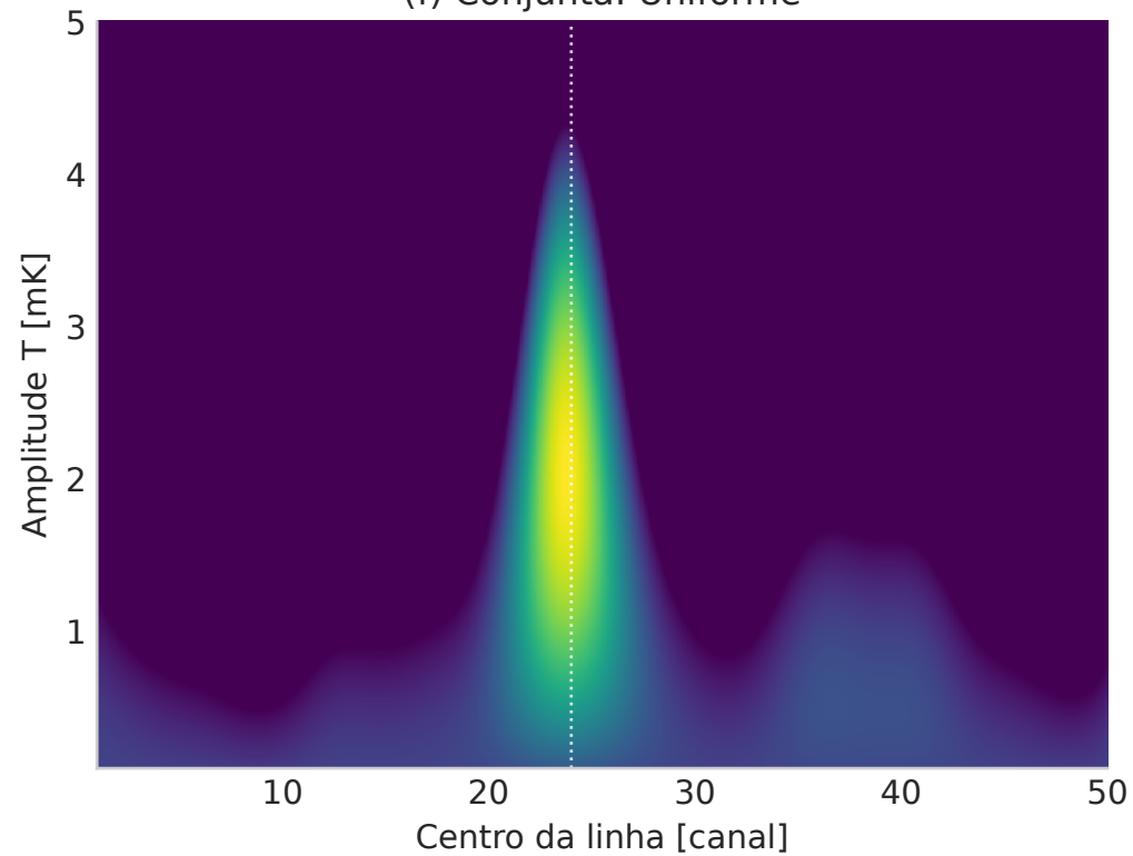
(f) Conjunta: Uniforme
