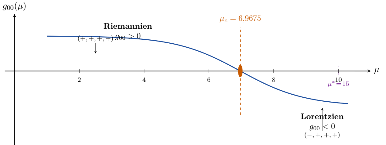
Figure 19.2 – Transition de signature lorentzienne. La composante métrique g_{00}(\mu) = -d^2(\ln \alpha_{\text{EM}})/d\mu^2 change de signe à l'échelle critique \mu_c = 6,9675 . Pour \mu > \mu_c (y compris \mu^* = 15 ), la géométrie de Fisher acquiert la signature lorentzienne (-, +, +, +) : le temps émerge de la courbure d'information.
