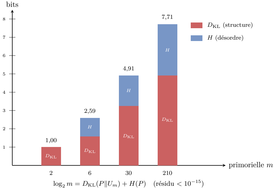
Figure 4.1 – Budget d'information du crible aux niveaux primoriels. La capacité totale \log_2 m (hauteur de la barre) est exactement partitionnée en structure ( D_{\text{KL}} , rouge) et désordre ( H , bleu) par l'identité GFT. Au fur et à mesure que m grandit, D_{\text{KL}} domine : le crible impose un ordre croissant.
