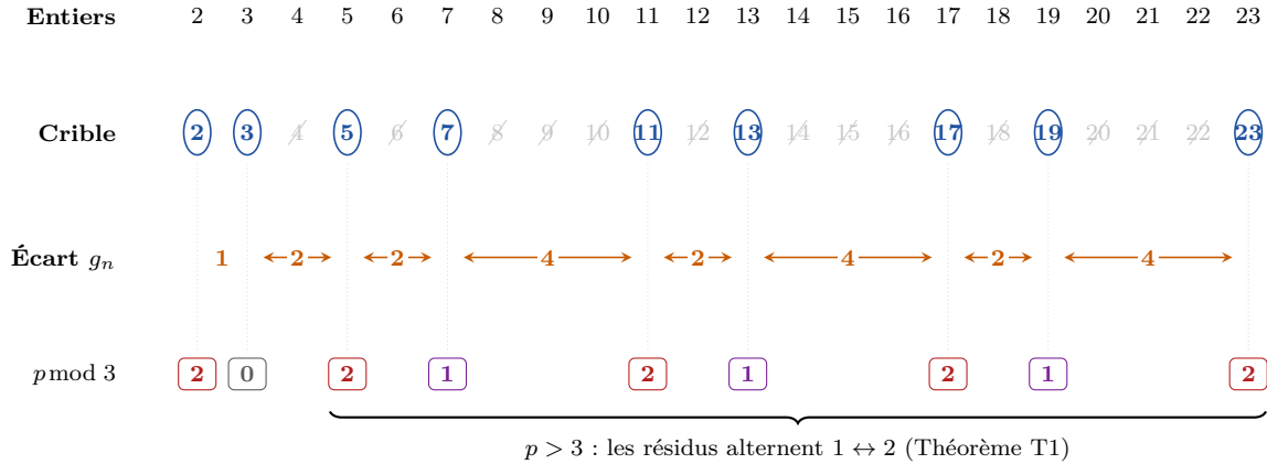
Figure 1.1 — Le processus de crible visualisé. Ligne 1 : entiers 2–23. Ligne 2 : composés rayés (Ératosthène), premiers encerclés. Ligne 3 : écarts g_n = p_{n+1} - p_n . Ligne 4 : résidus mod 3—après p = 3 , ils alternent strictement entre 1 et 2, interdits de se répéter (T1).
