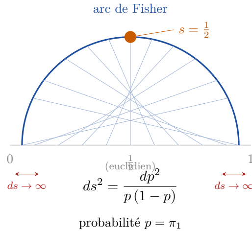
Figure 5.1 – Métrique de Fisher sur le simplexe binaire \Delta_2 . L'intervalle euclidien [0, 1] (gris) est « courbé » par la métrique de Fisher ds^2 = dp^2 / [p(1 - p)] en un demi-cercle (arc bleu). Les lignes de grille relient des valeurs de probabilité égales : elles se resserrent près des bords ( p \rightarrow 0 ou p \rightarrow 1 ), montrant la divergence de la métrique. Le point stationnaire s = 1/2 (orange) se trouve au milieu géodésique. C'est l'unique métrique monotone sur \Delta_2 (Čencov).
