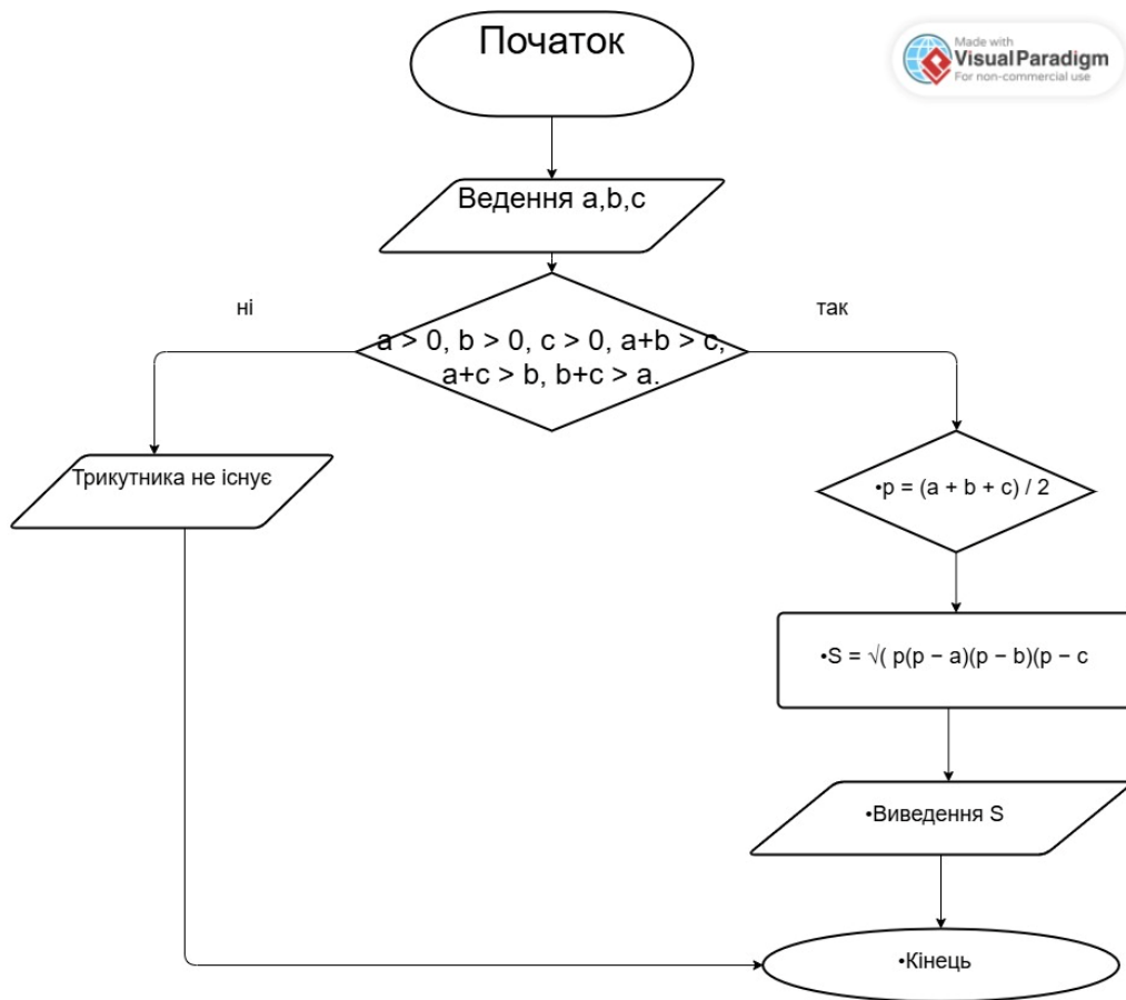
Рис. 1. Алгоритм програми обчислення площі трикутника за трьома сторонами
