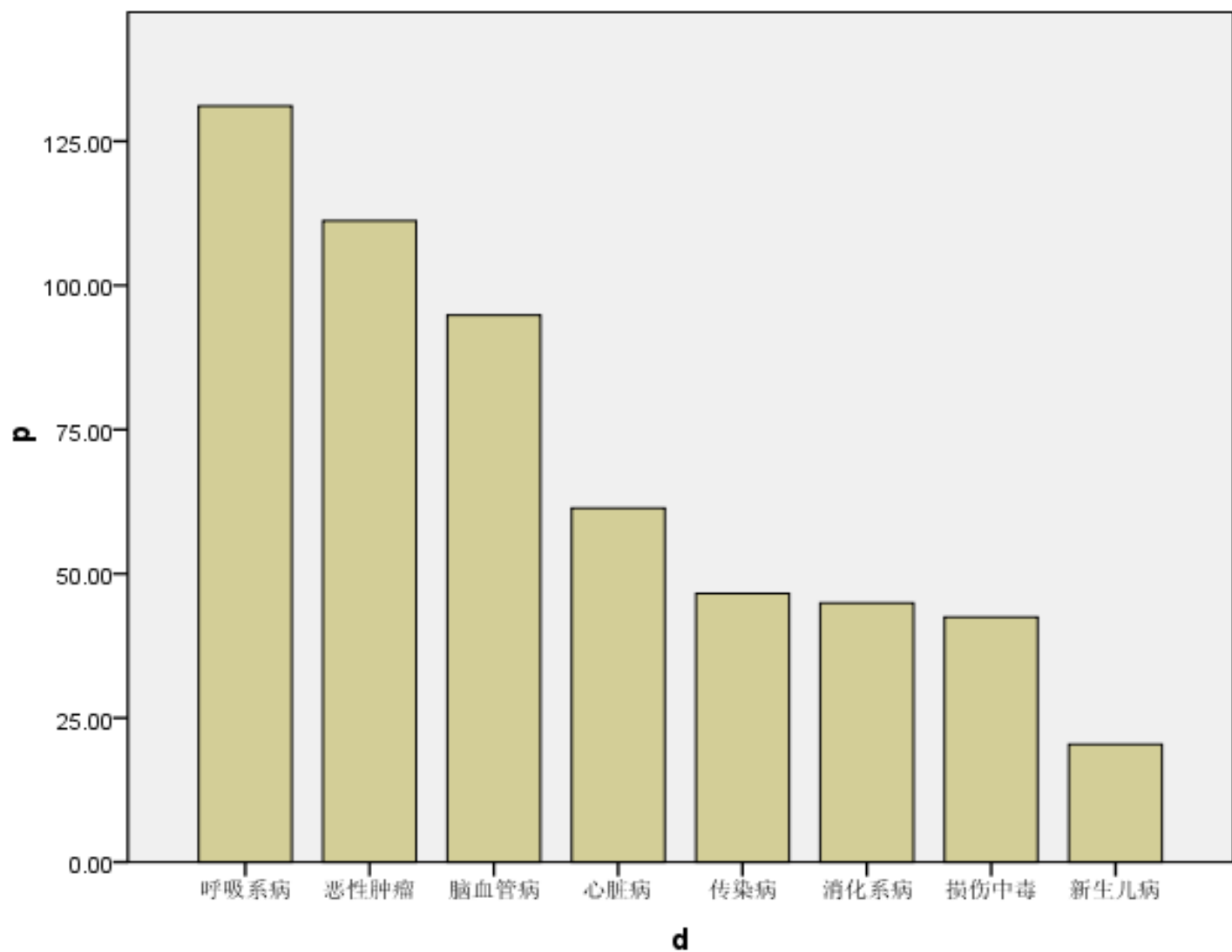
图10-1 某年某地主要死因的死亡率（1/10万）
