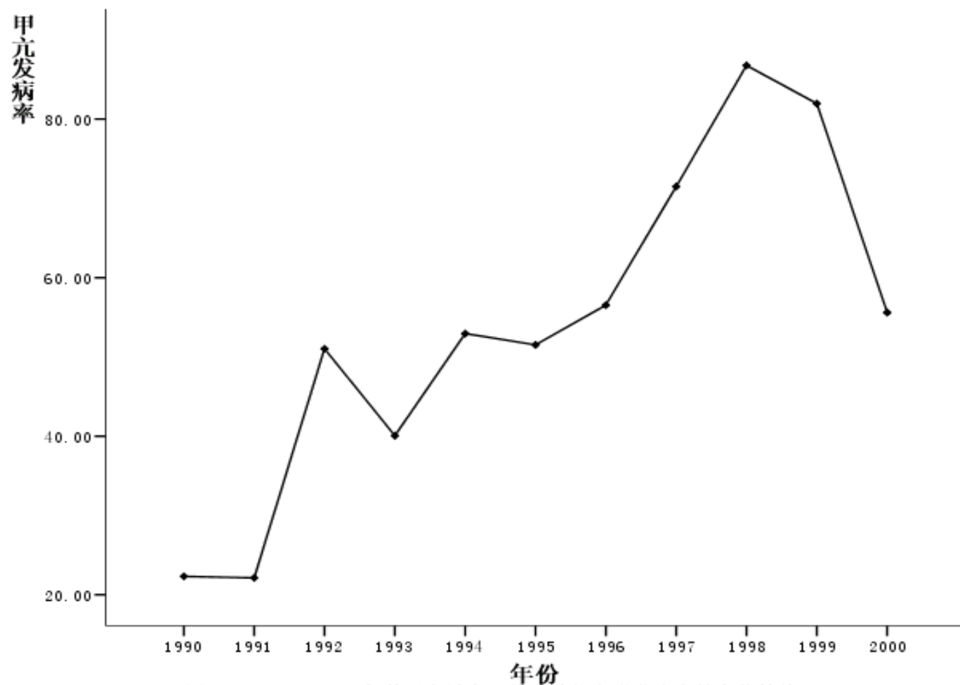
图10-4 1990-2000年某沿海城市甲状腺功能亢进发病率的变化趋势
