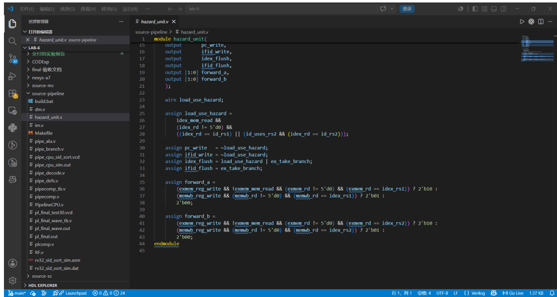
图 2: 流水线 CPU 中 forward_a 与 forward_b 的 RAW 数据转发判断
