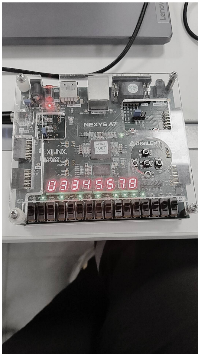
图 14: 测试 5: 开发板上流水线 CPU 运行学号排序程序
