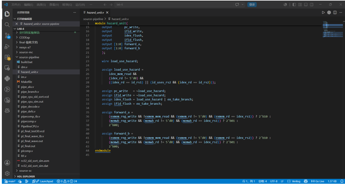
图 3: 流水线 CPU 的 load-use 冒险检测、暂停和 bubble 插入
