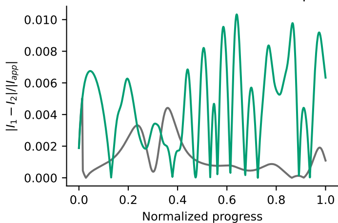
10% LLI+LAMn vs +10% LAMP
