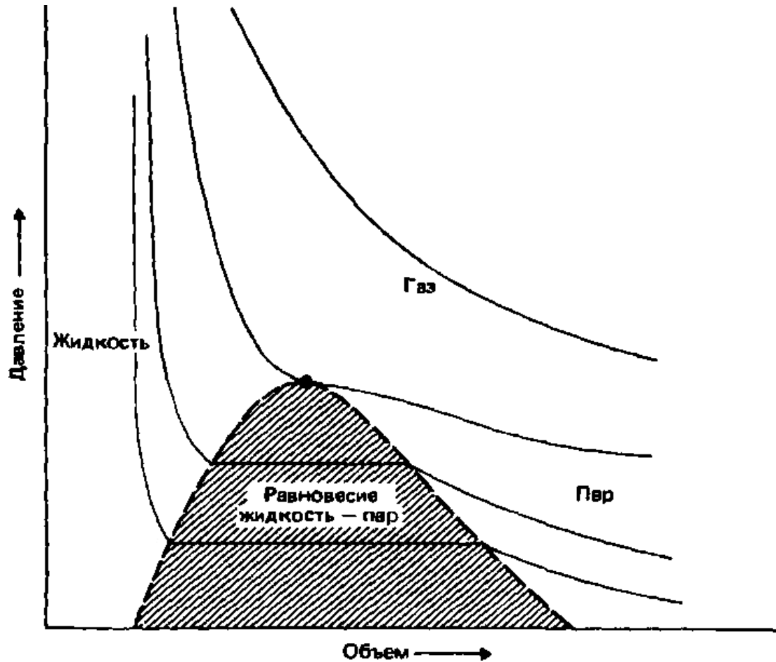
Рис. 10: Изотермы Эндрюса
