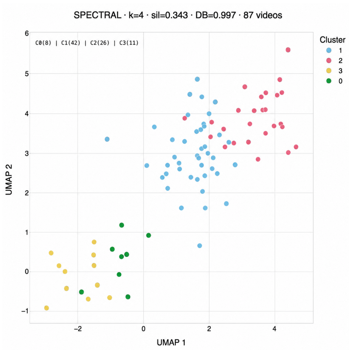
Рисунок 12 – Пример результата кластеризации видео
