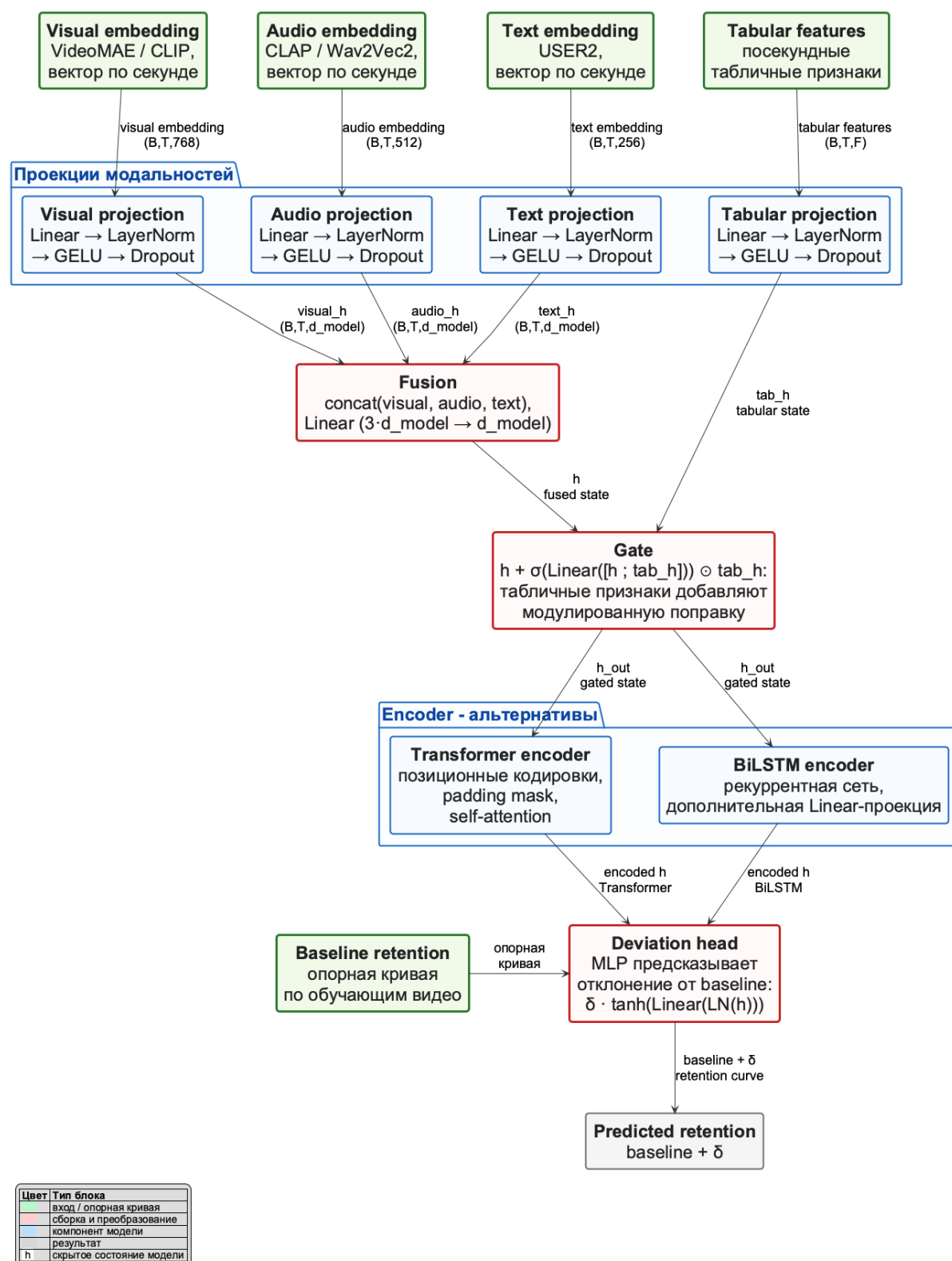
Рисунок 17 – Архитектура мультимодальной модели удержания с объединением модальностей и табличным гейтом
