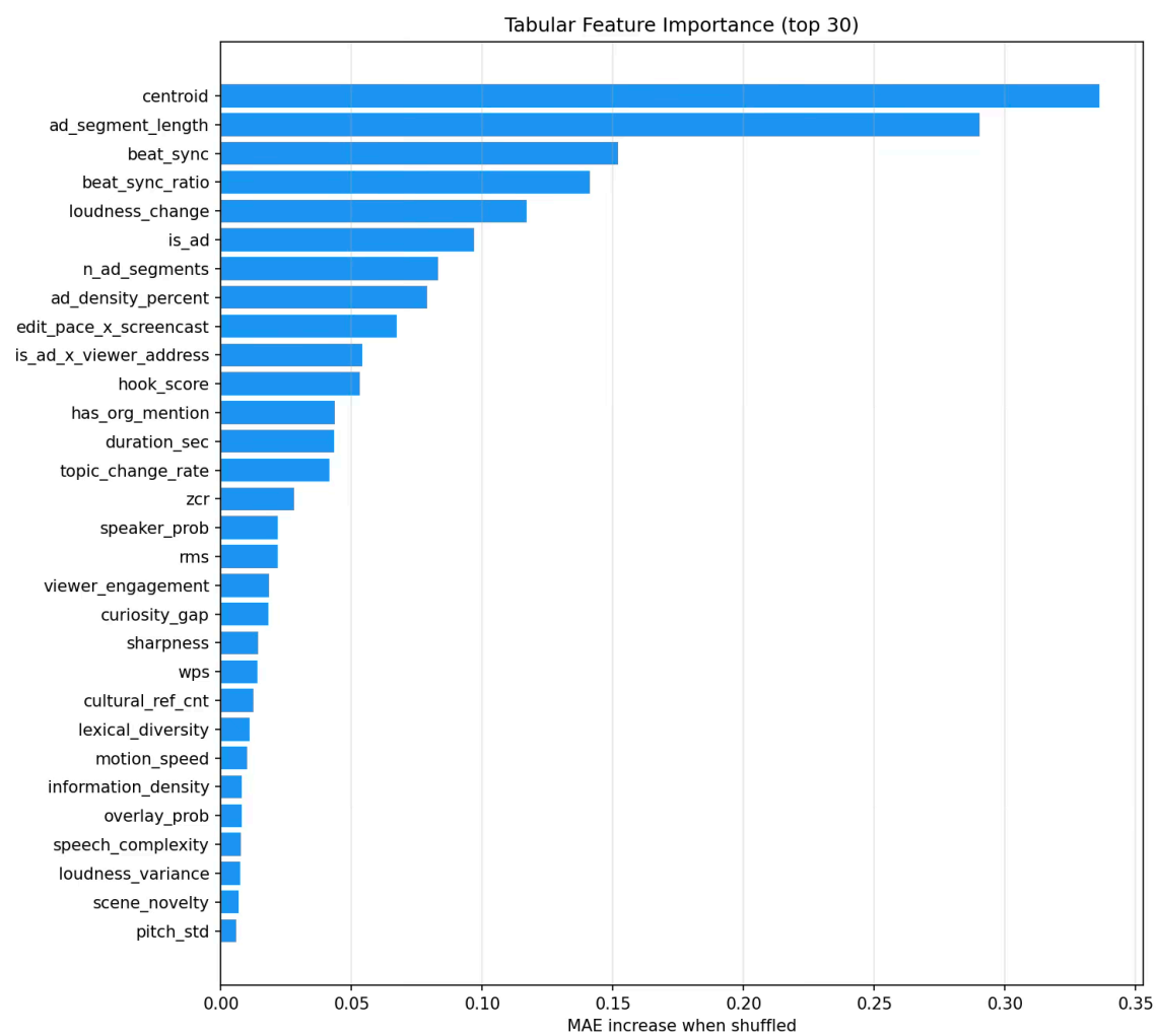
Рисунок 14 – Дополнительный пример визуализации значимости признаков
