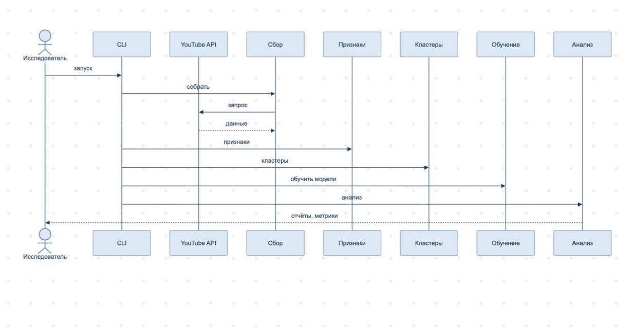
Рисунок 1 – Последовательность выполнения основных этапов пайплайна
