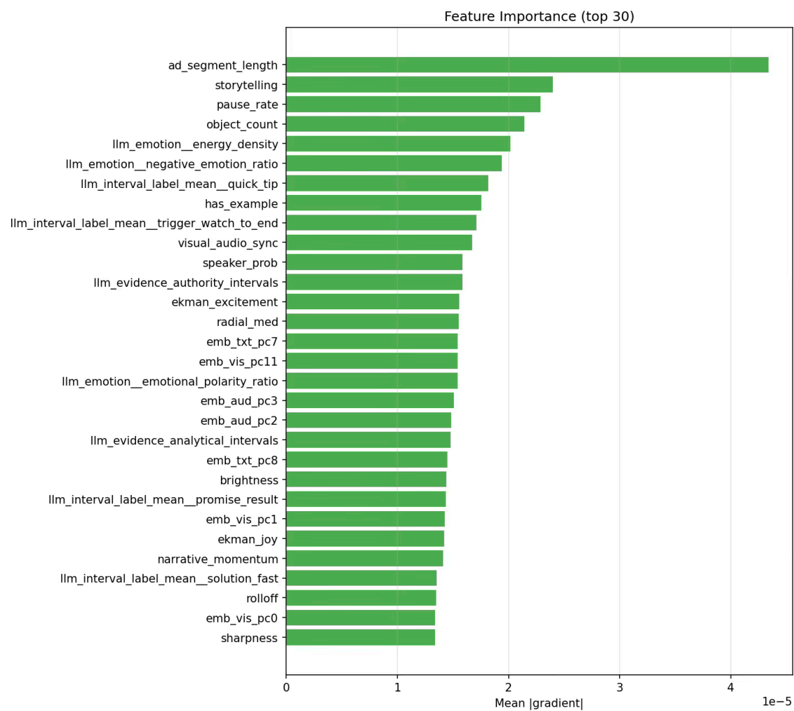
Рисунок 13 – Пример визуализации значимости признаков
