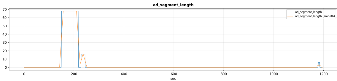
Рисунок 4 – Посекундный признак длины рекламного сегмента ( ad_segment_length ) и его сглаженная версия
