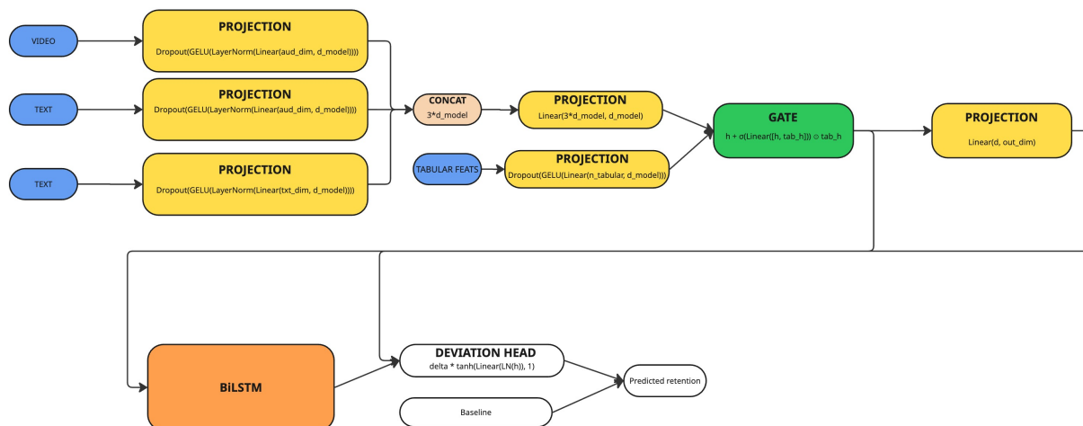
Рисунок 8 – Схема мультимодальной рекуррентной (LSTM) архитектуры прогнозирования удержания
