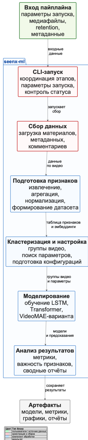
Рисунок 15 – Контейнерная архитектура пайплайна seenx-ml (C4 L2)
