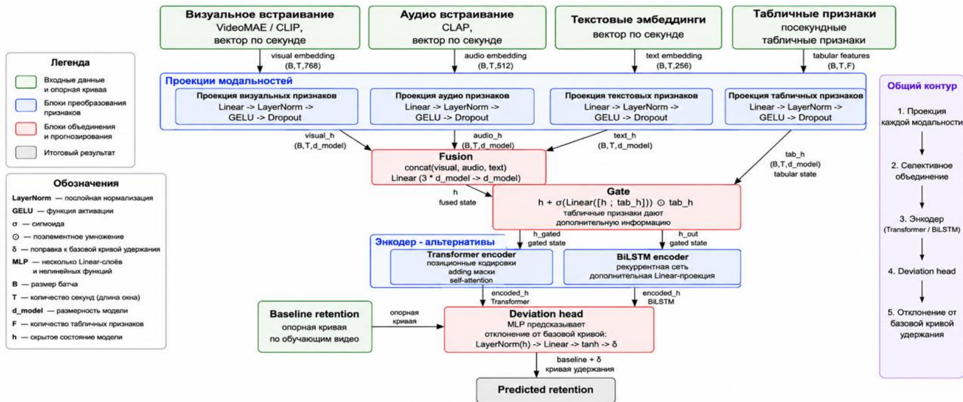
Рисунок 18 – Архитектура мультимодальной модели удержания с объединением модальностей и табличным гейтом: более полный вариант
