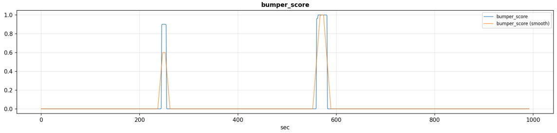
Рисунок 1 – Посекундный признак вероятности заставки (bumper_score) и его сглаженная версия
