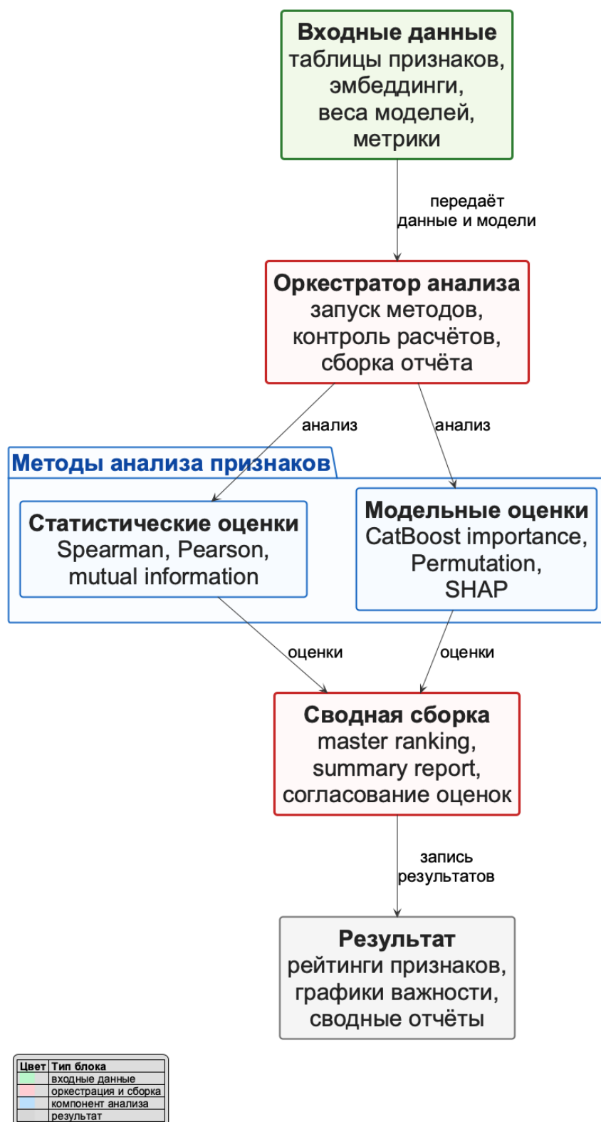
Рисунок 17 – Схема анализа значимости признаков и формирования сводных отчётов (C4 L3)
