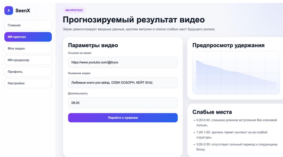
Рисунок 19 – Экран ввода параметров видео и предпросмотра прогноза удержания
