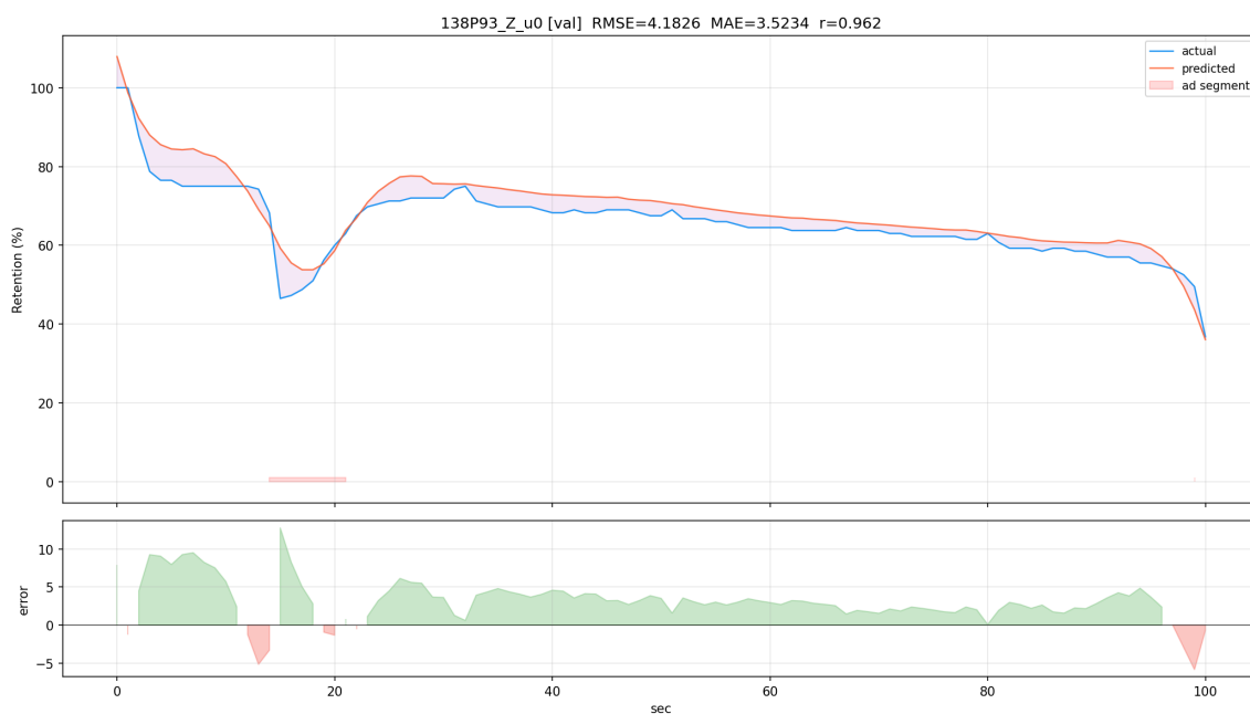
Рисунок 9 – Пример предсказания Transformer для второго валидационного видеоролика
