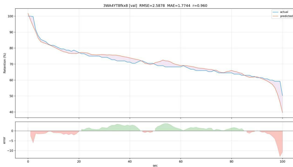
Рисунок 8 – Пример предсказания Transformer для первого валидационного видеоролика
