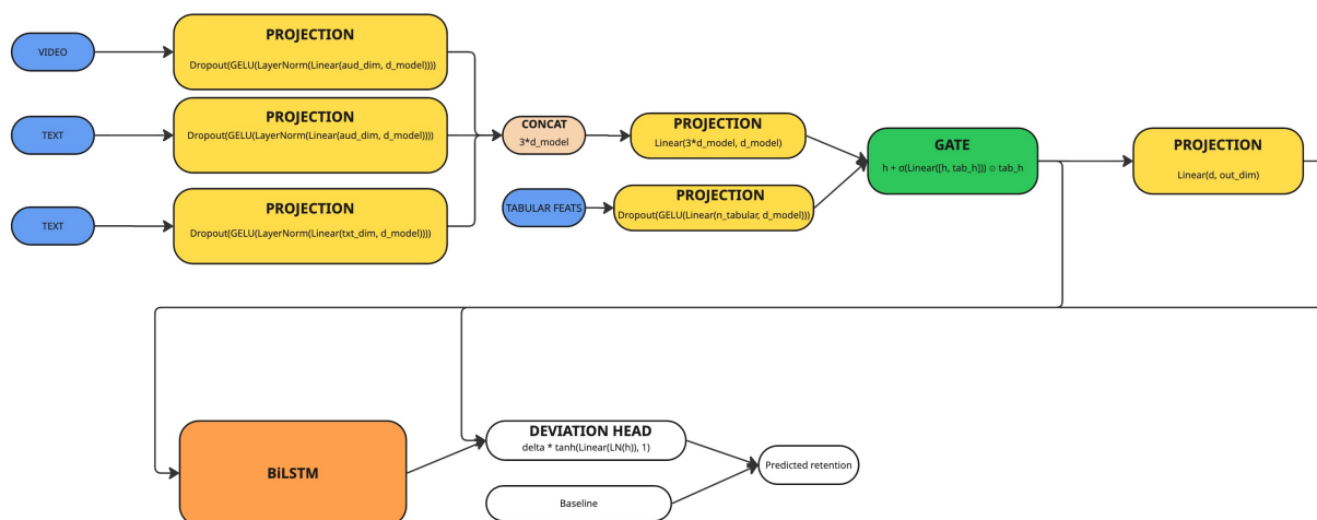
Рисунок 7 – Схема мультимодальной рекуррентной (LSTM) архитектуры прогнозирования удержания
