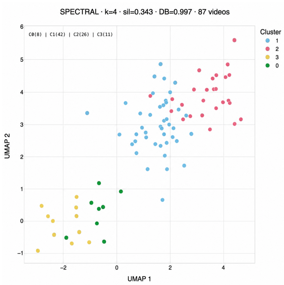
Рисунок 11 – Пример результата кластеризации видео
