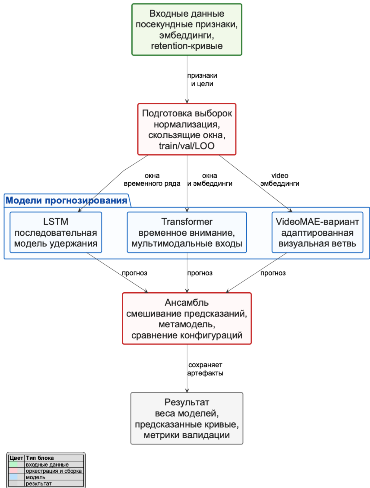
Рисунок 15 – Общая схема архитектур прогнозирования удержания зрителей
