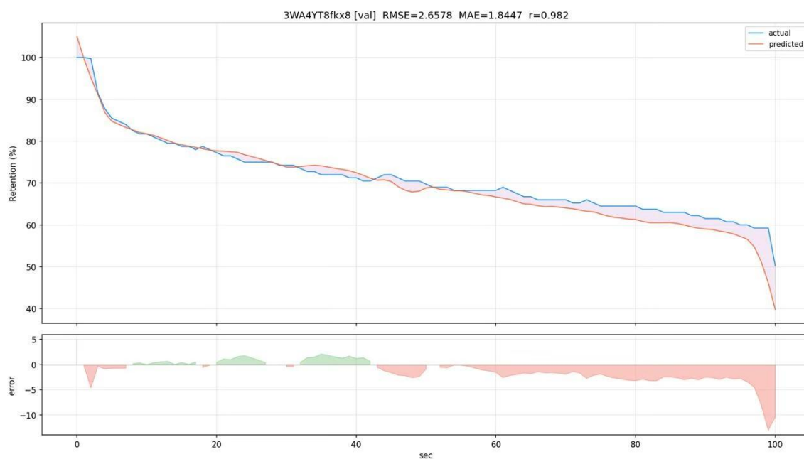
Рисунок 10 – Пример предсказания Transformer для третьего валидационного видеоролика
