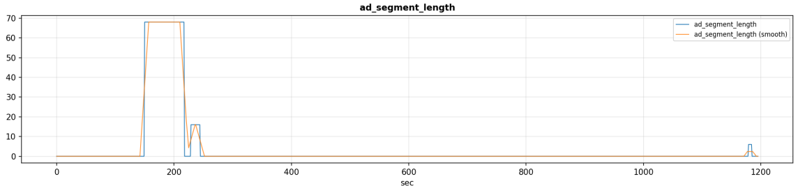
Рисунок 3 – Посекундный признак длины рекламного сегмента (ad_segment_length) и его сглаженная версия
