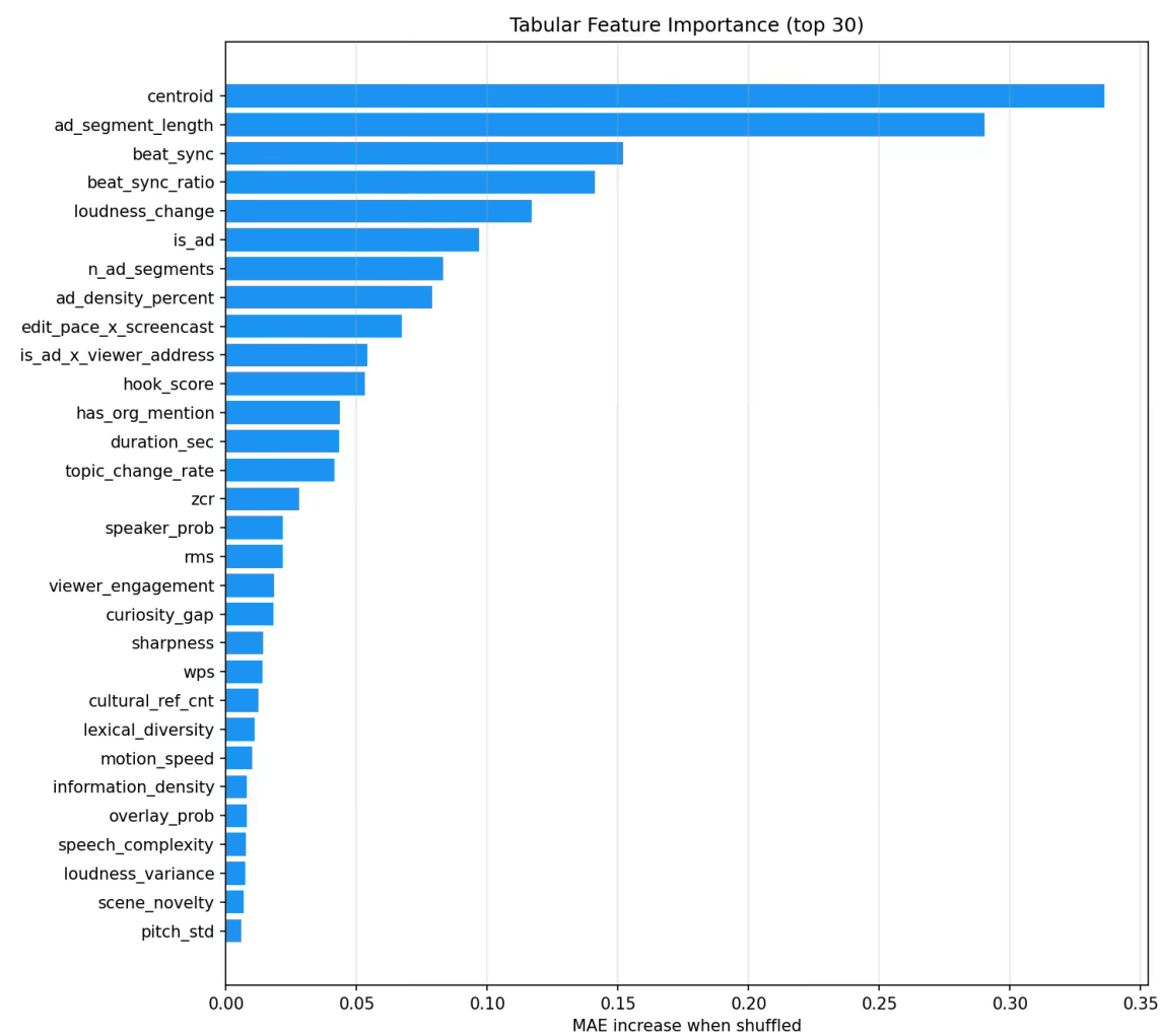
Рисунок 13 – Дополнительный пример визуализации значимости признаков
