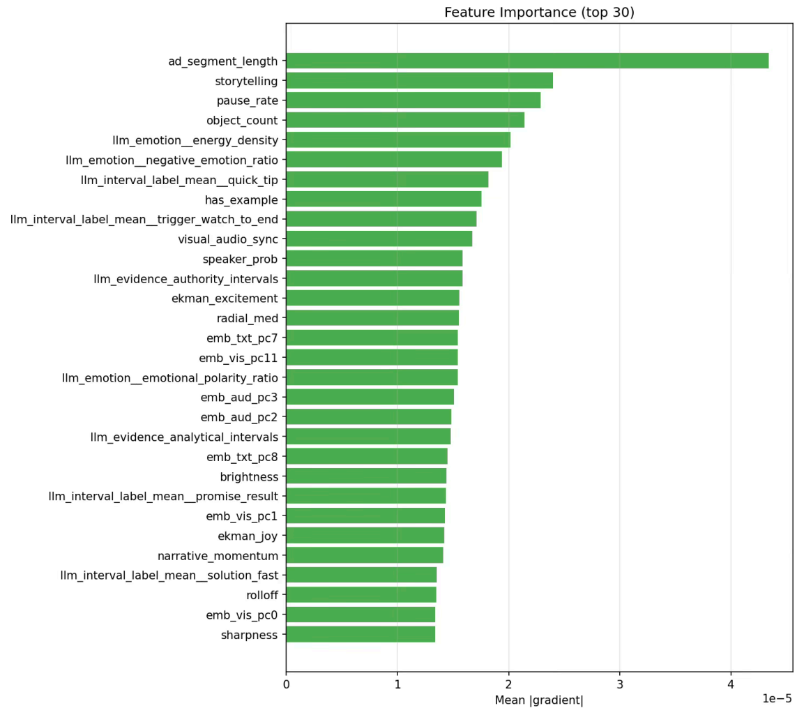
Рисунок 12 – Пример визуализации значимости признаков
