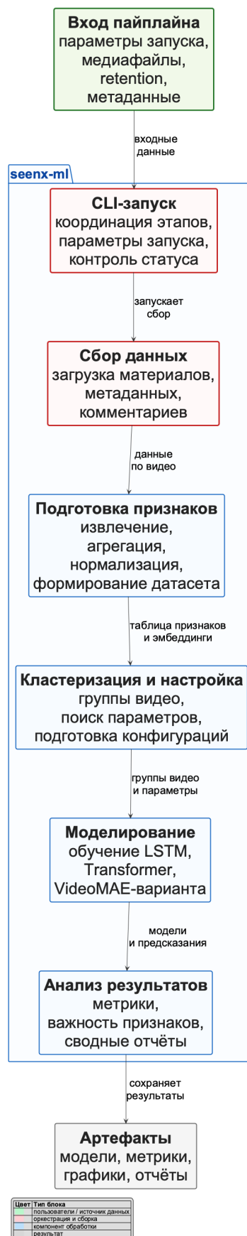
Рисунок 14 – Контейнерная архитектура пайплайна seenx-ml (C4 L2)
