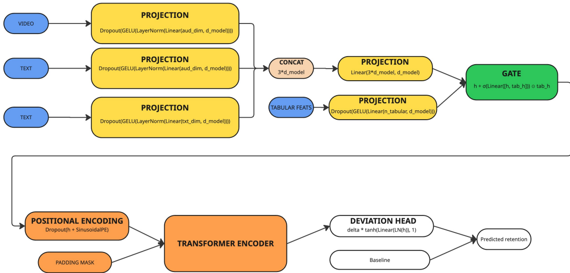
Рисунок 6 – Схема мультимодальной трансформерной архитектуры прогнозирования удержания
