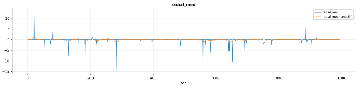
Рисунок 4 — Медианная радиальная компонента оптического потока ( radial_med ) и её сглаженная версия
