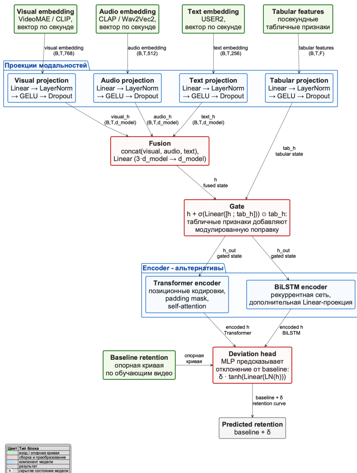
Рисунок 17 – Архитектура мультимодальной модели удержания с объединением модальностей и табличным гейтом (C4 L2)
