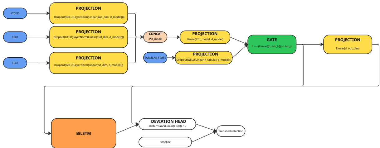
Рисунок 7 – Схема мультимодальной рекуррентной (LSTM) архитектуры прогнозирования удержания
