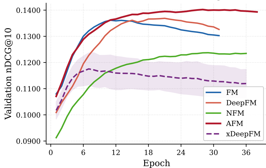
BGG — Validation nDCG@10
