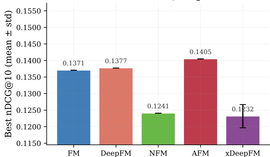
BGG — Best nDCG@10 per Model
