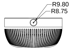
vista posteriore
