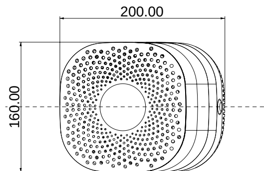
vista superiore
