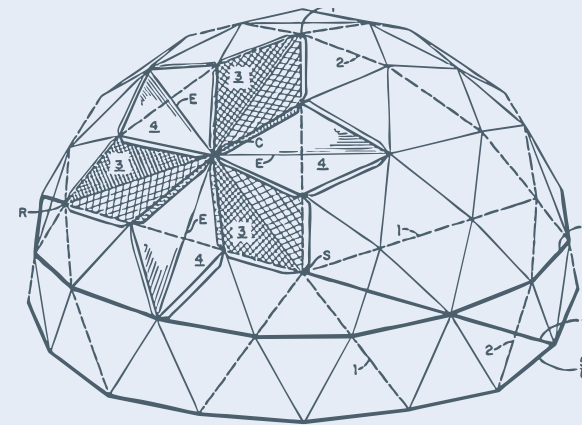
Geodätische Kuppel, Buckminster Fuller – 1965 Grundmuster als räumliches Bezugssystem
