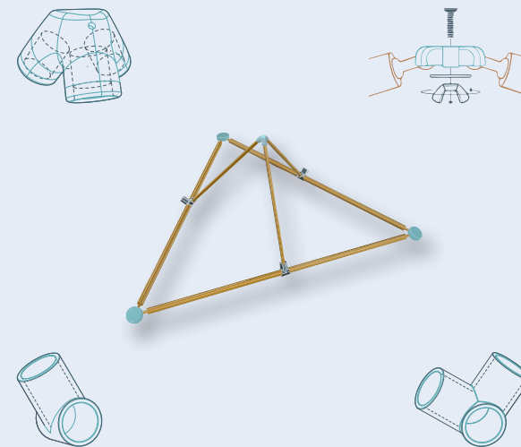
Pavillonmodul: 3D-gedruckte Verbindungs-Elementen Grundstruktur aus Stäben und Knotenpunkten
