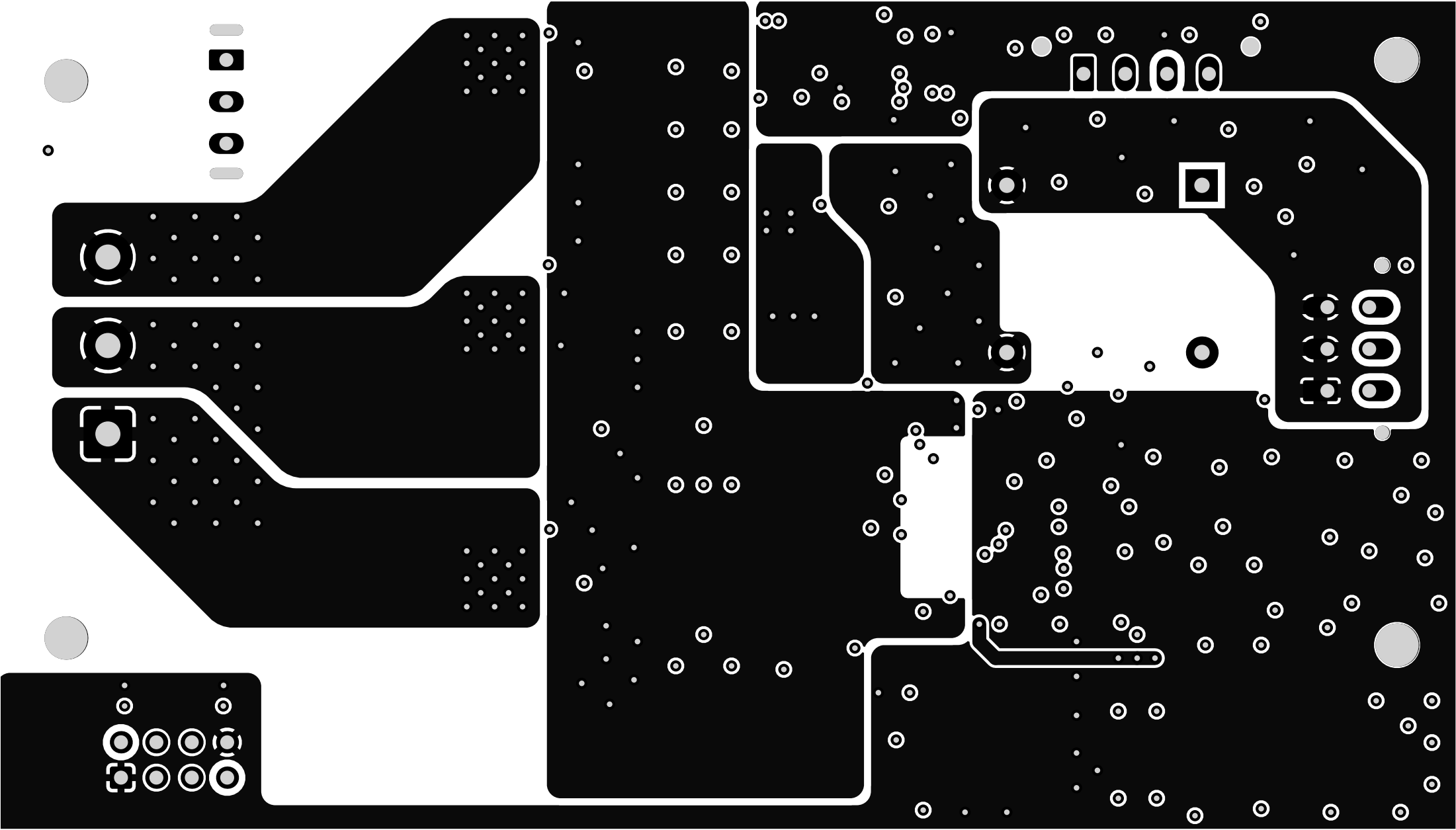
VCC Layer
