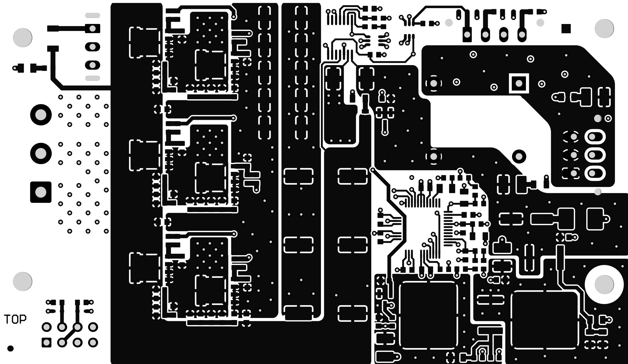
Top Layer
