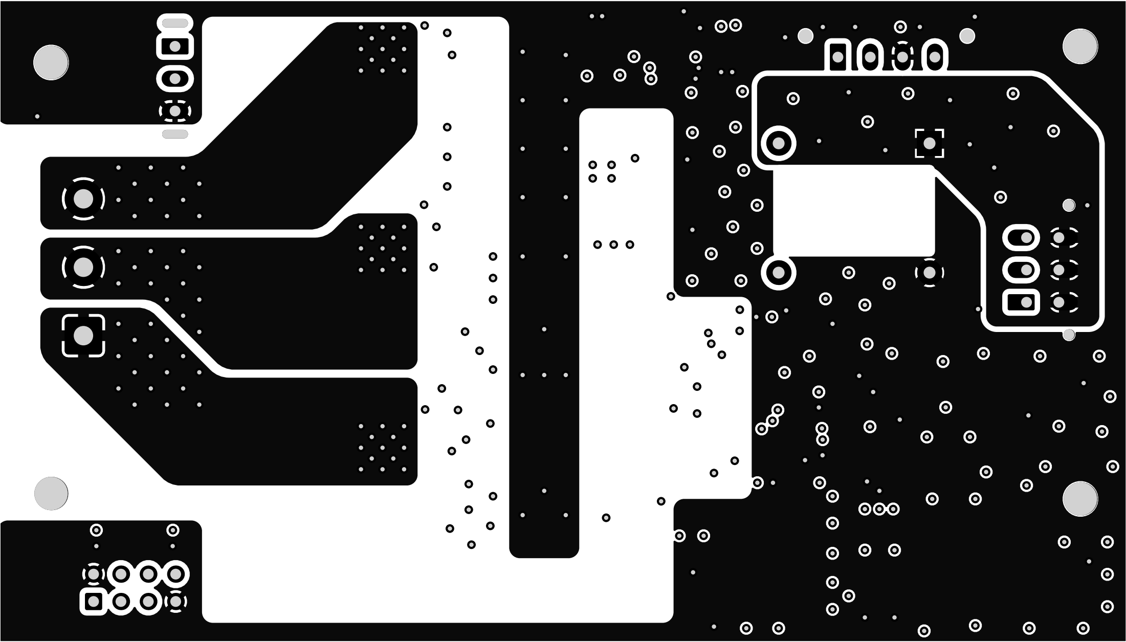
GND Layer
