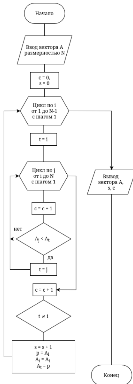
Рисунок 13 – Блок-схема алгоритма сортировки выбором
