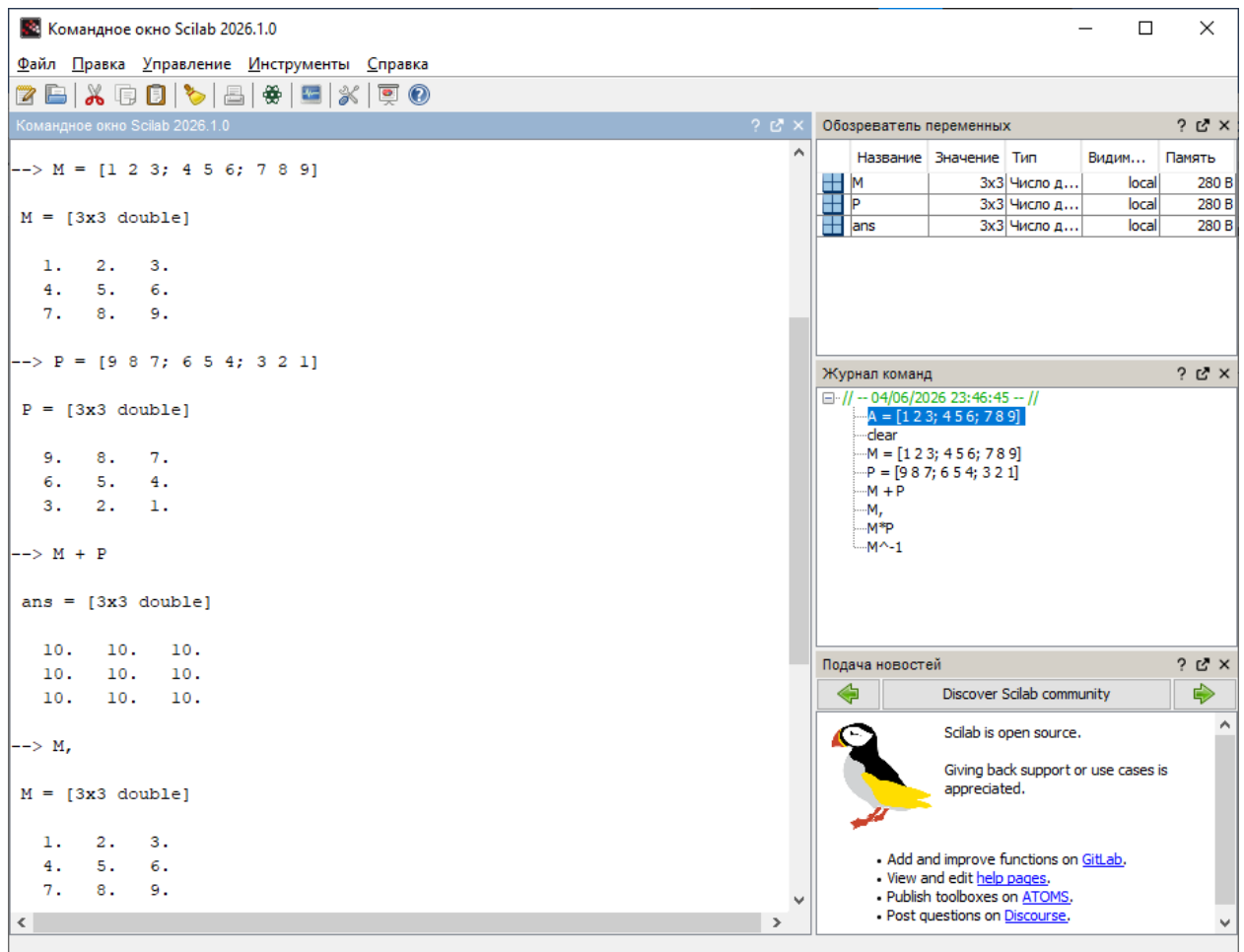
Рисунок 7а – Математические операции с матрицами в Scilab
