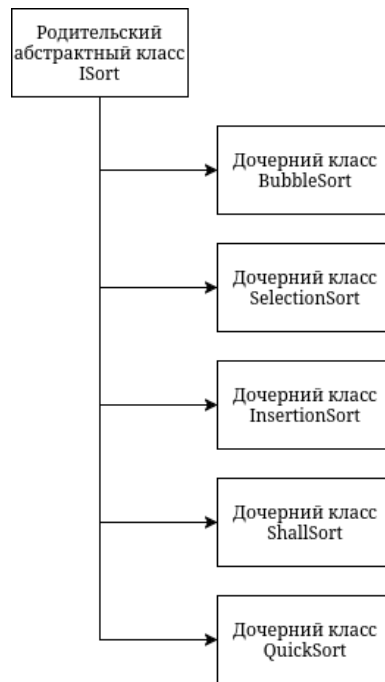
Рисунок 19 – Структура наследования классов сортировки
