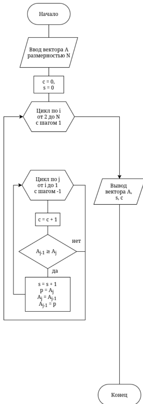
Рисунок 14 – Блок-схема алгоритма сортировки вставкой
