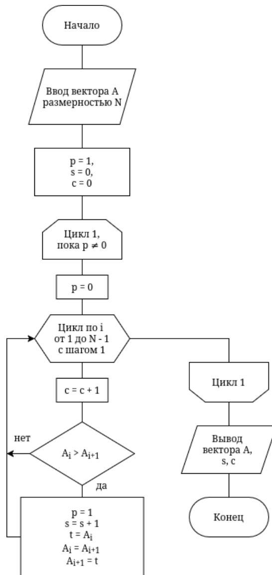
Рисунок 12 – Блок-схема алгоритма пузырьковой сортировки
