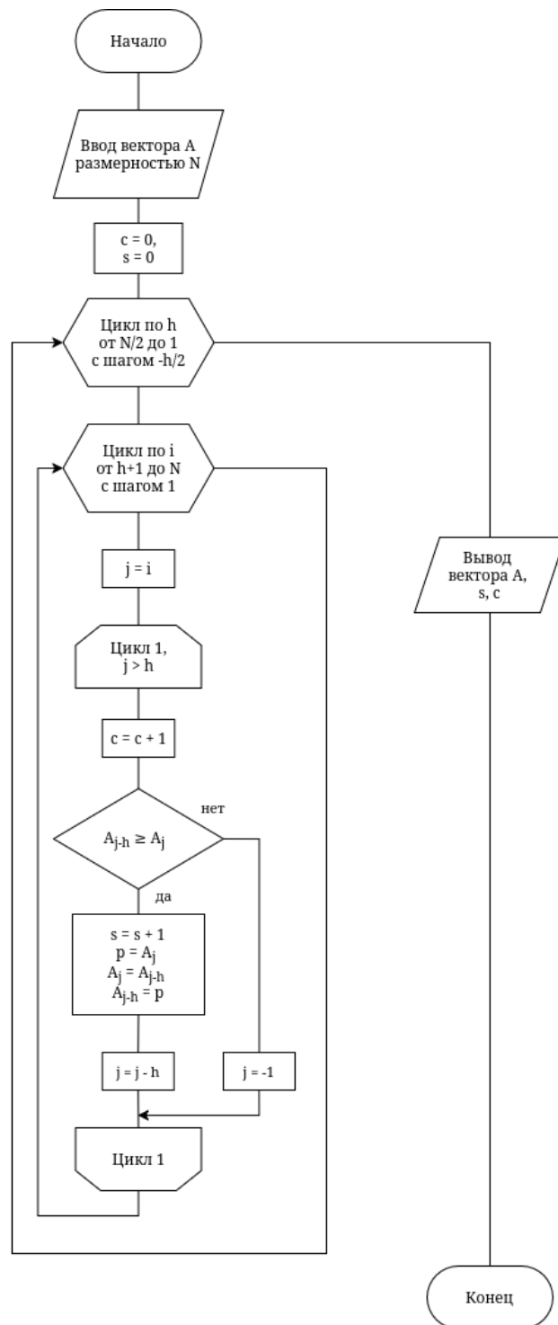
Рисунок 15 – Блок-схема алгоритма сортировки Шелла
