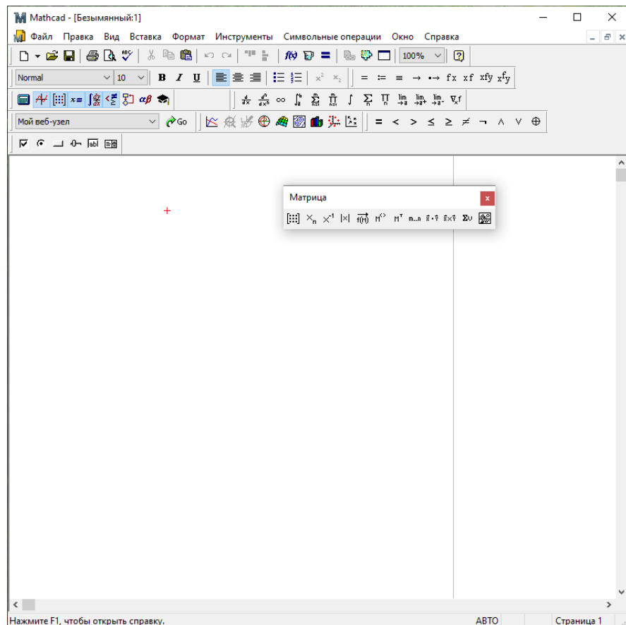
Рисунок 3 – Интерфейс Mathcad
