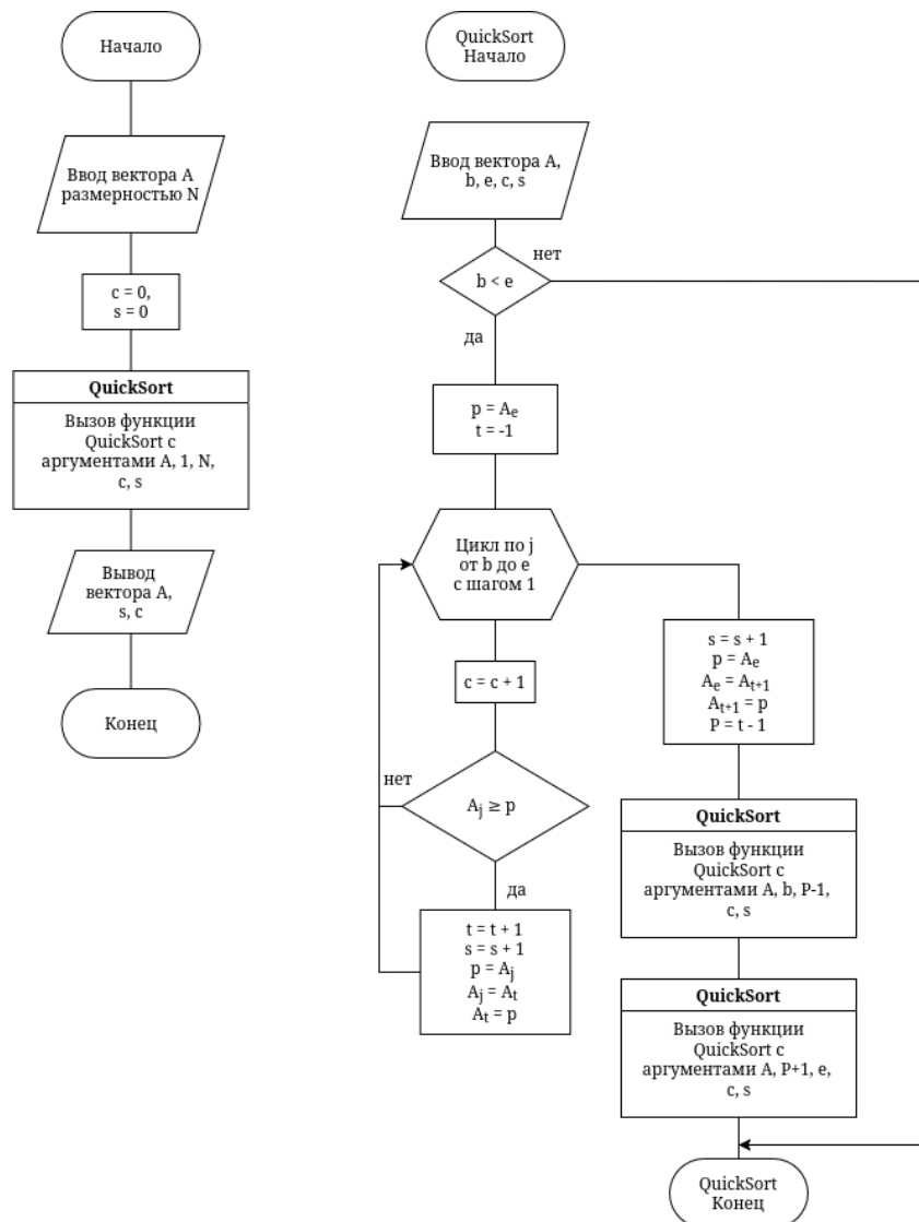
Рисунок 16 – Блок-схема алгоритма быстрой сортировки
