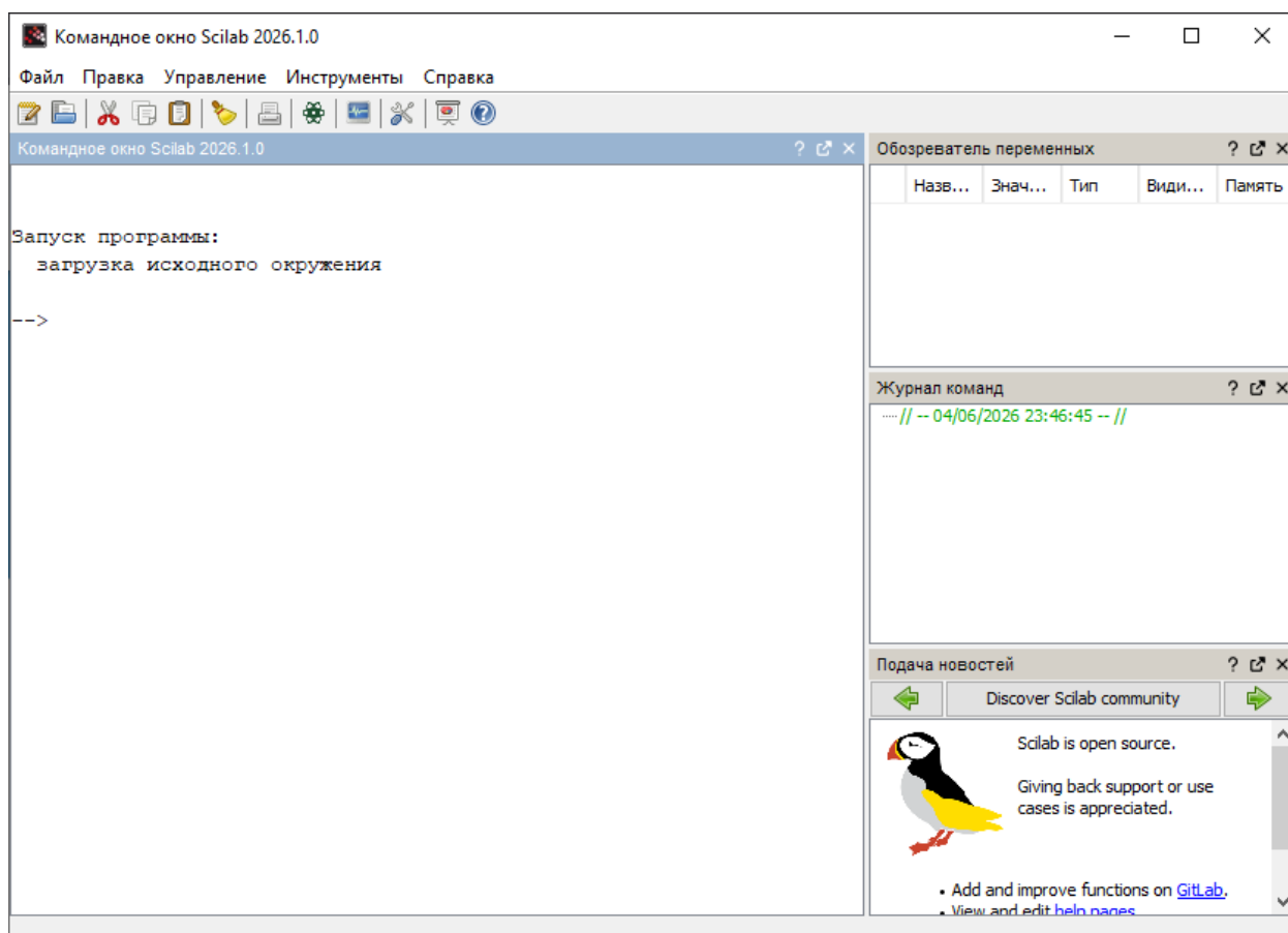
Рисунок 6 – Интерфейс Scilab
