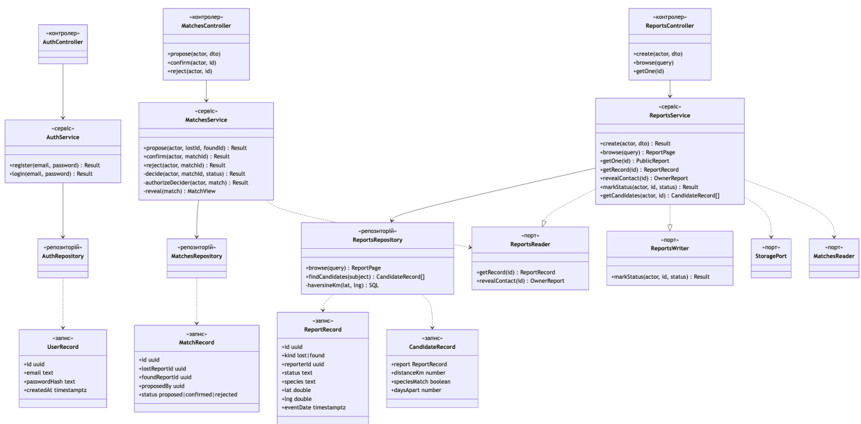
Рисунок 3.3 – Діаграма класів серверної частини
