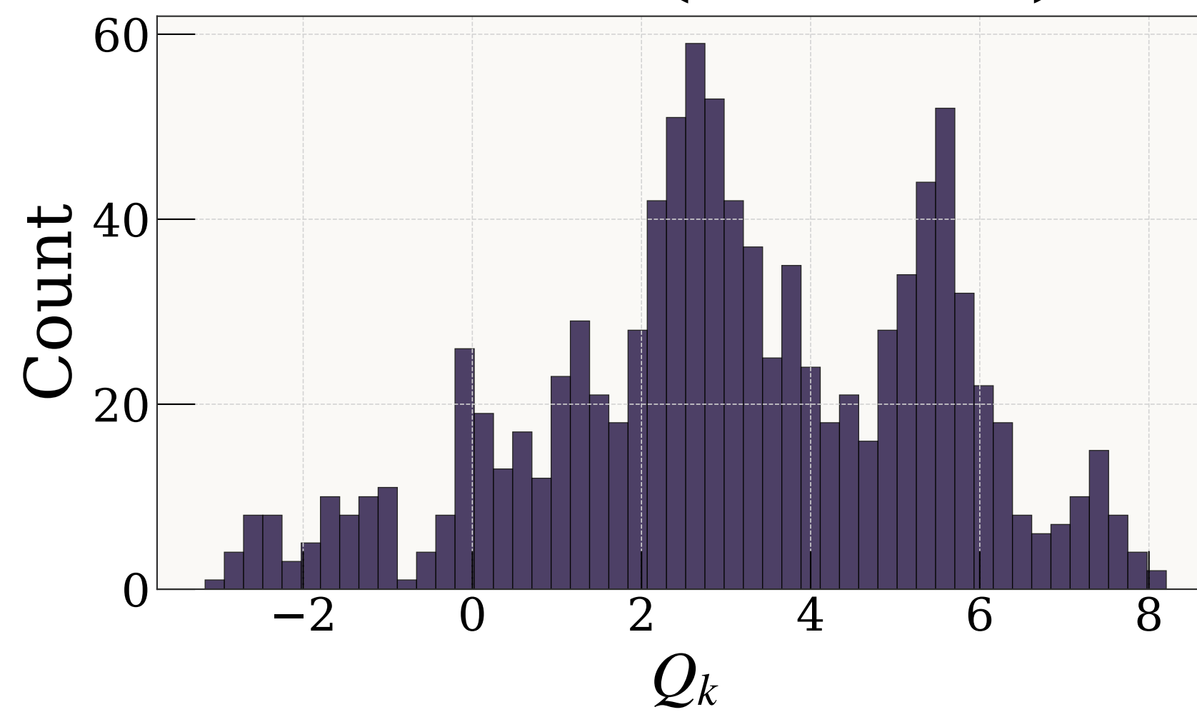
Mode 2 (-77 cm -1 )
