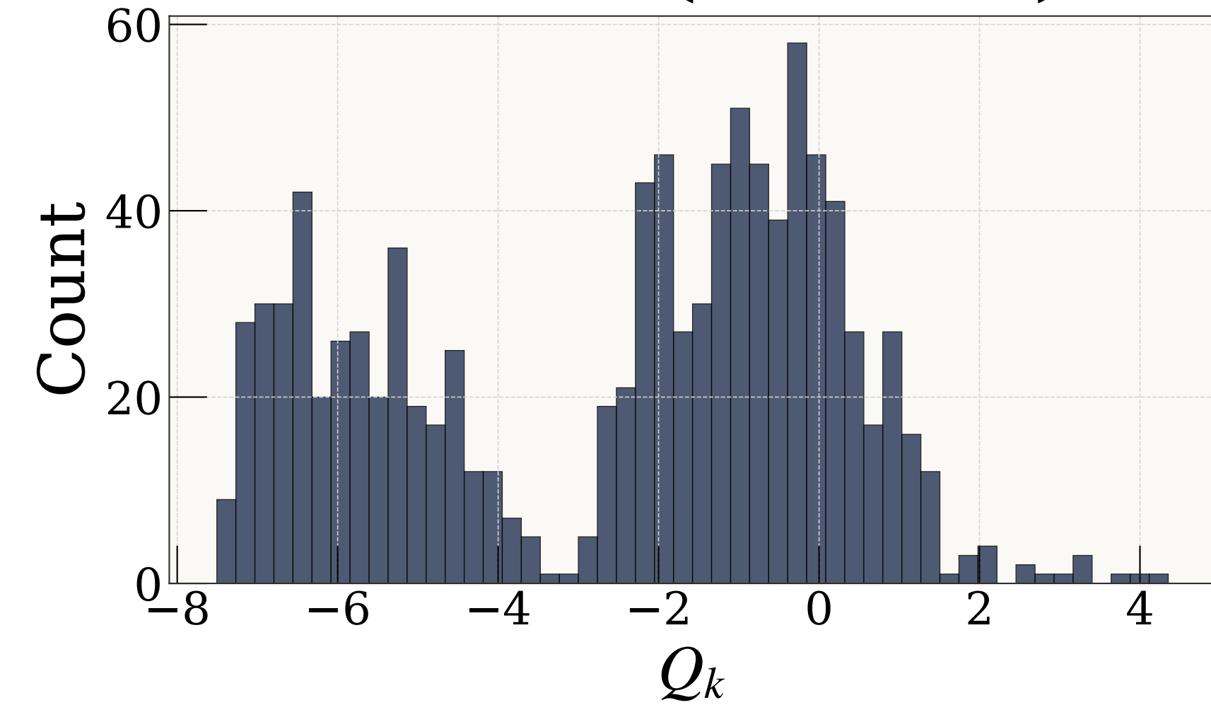
Mode 3 (-39 cm -1 )
