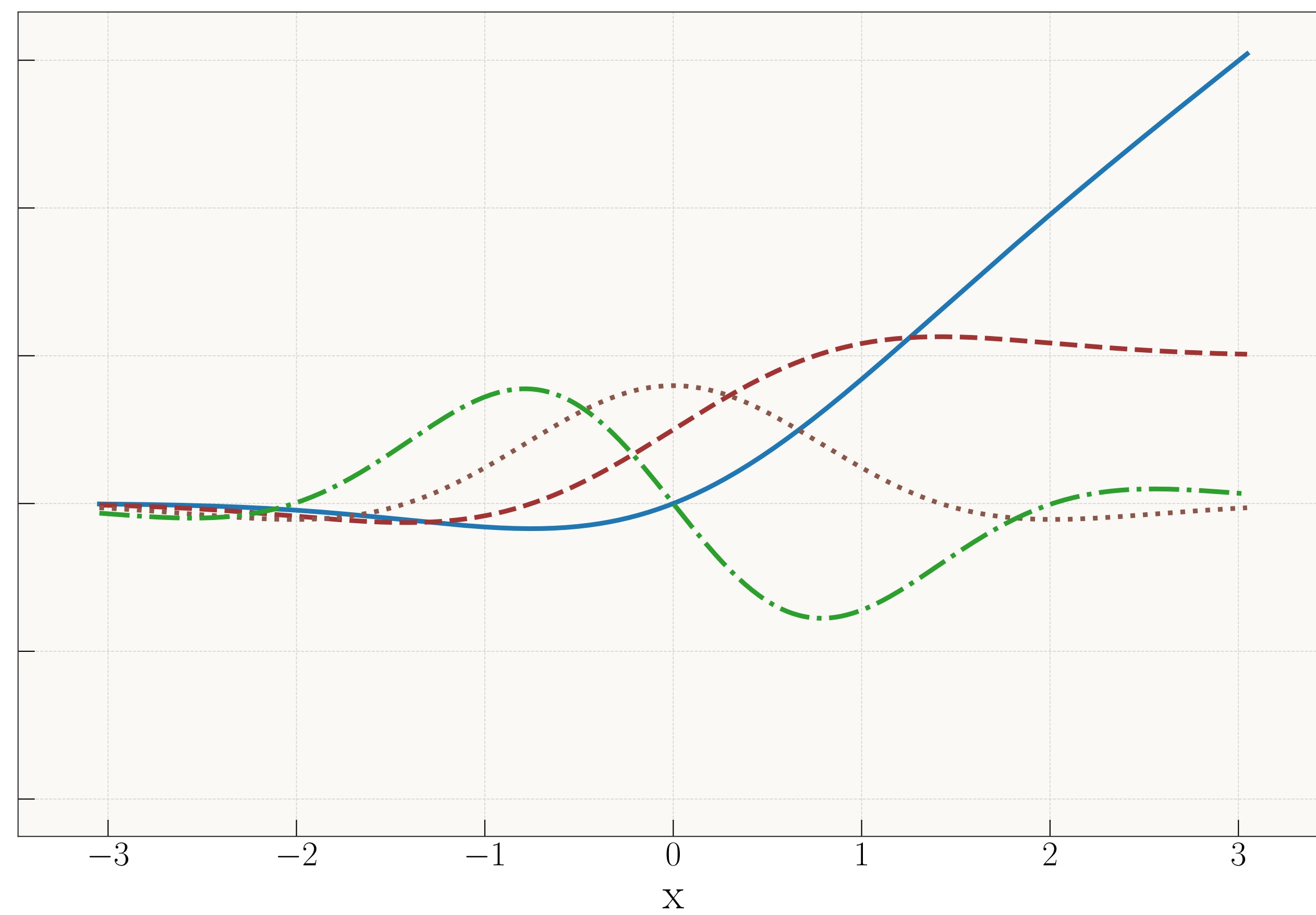
GELU
