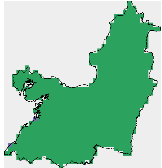
altitud – centro
