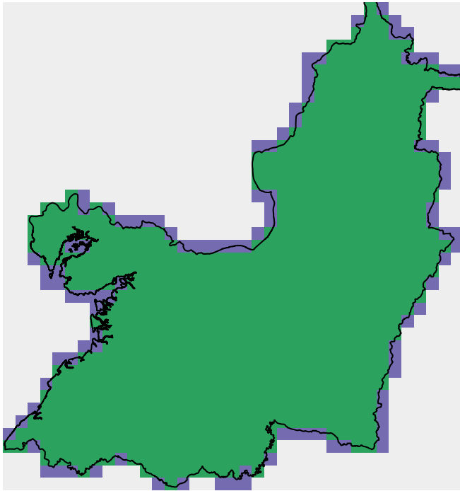
precipitacion – centro
