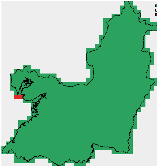
precipitacion – interseccion
