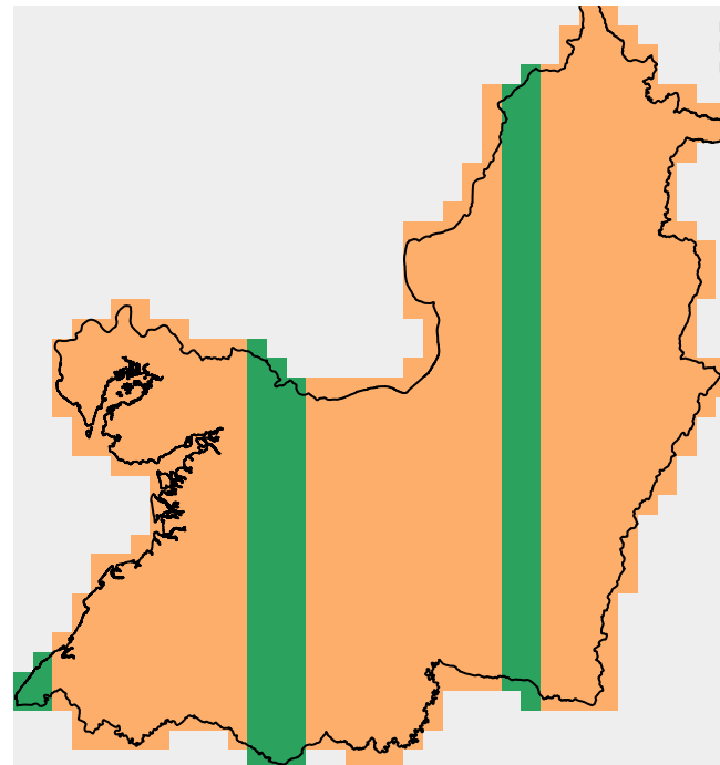
temperatura – interseccion
