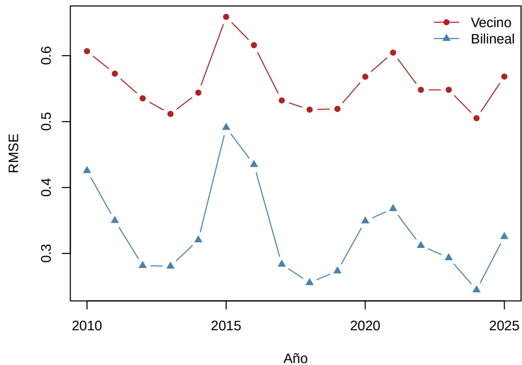
Comparación global temperatura
