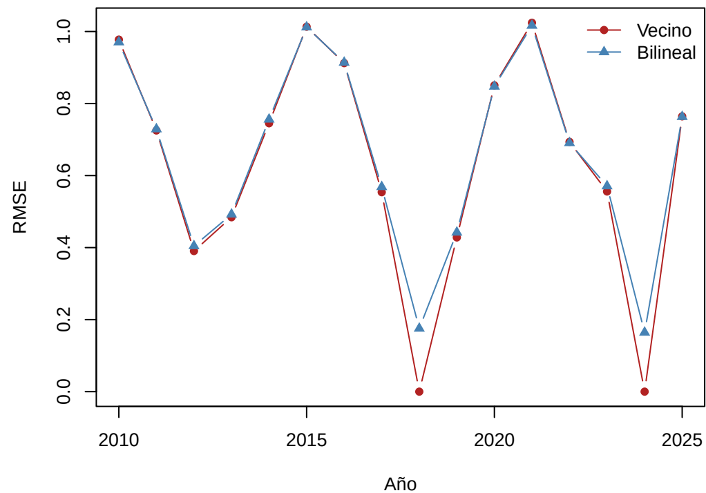
Comparación global radiacion
