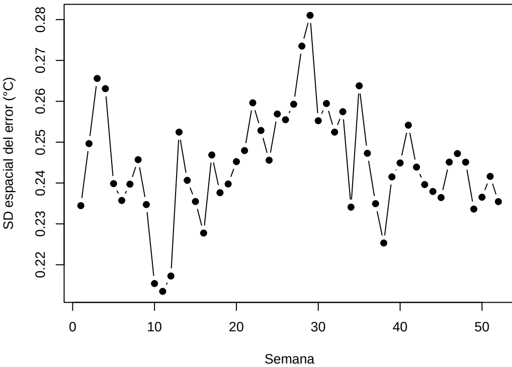
Error de temperatura por semana
