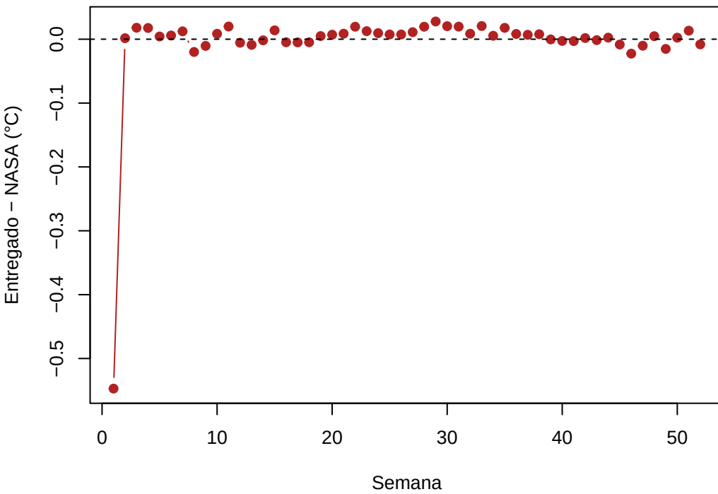
Sesgo medio semanal temperatura
