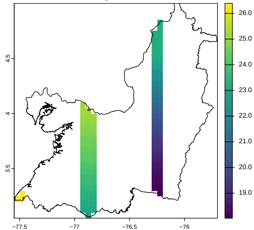
POWER: temperatura semanal
