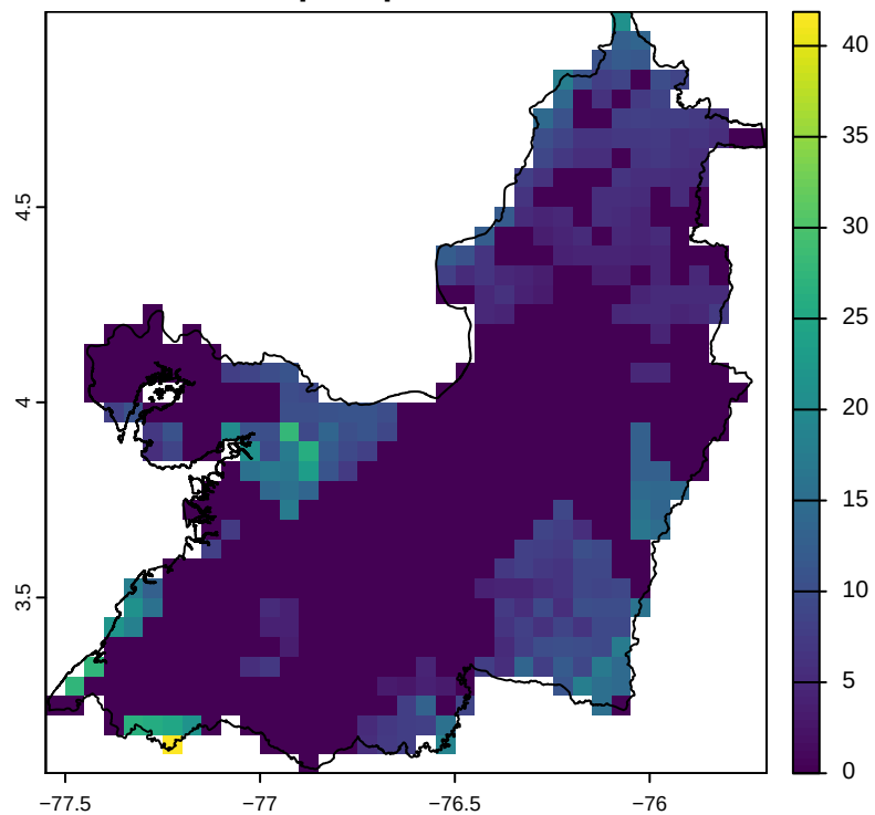
CHIRPS: precipitacion semanal
