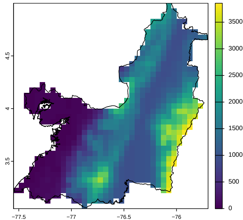
SRTM: altitud estatica
