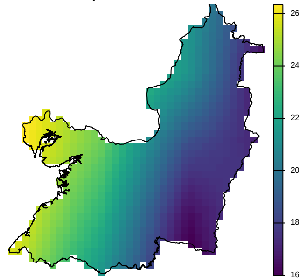
temperatura bilineal c
