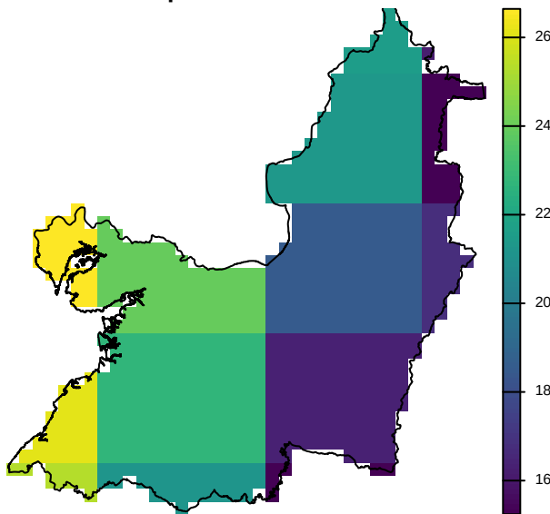
temperatura vecino c
