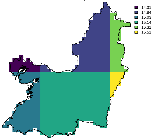
radiacion vecino mj m2 dia
