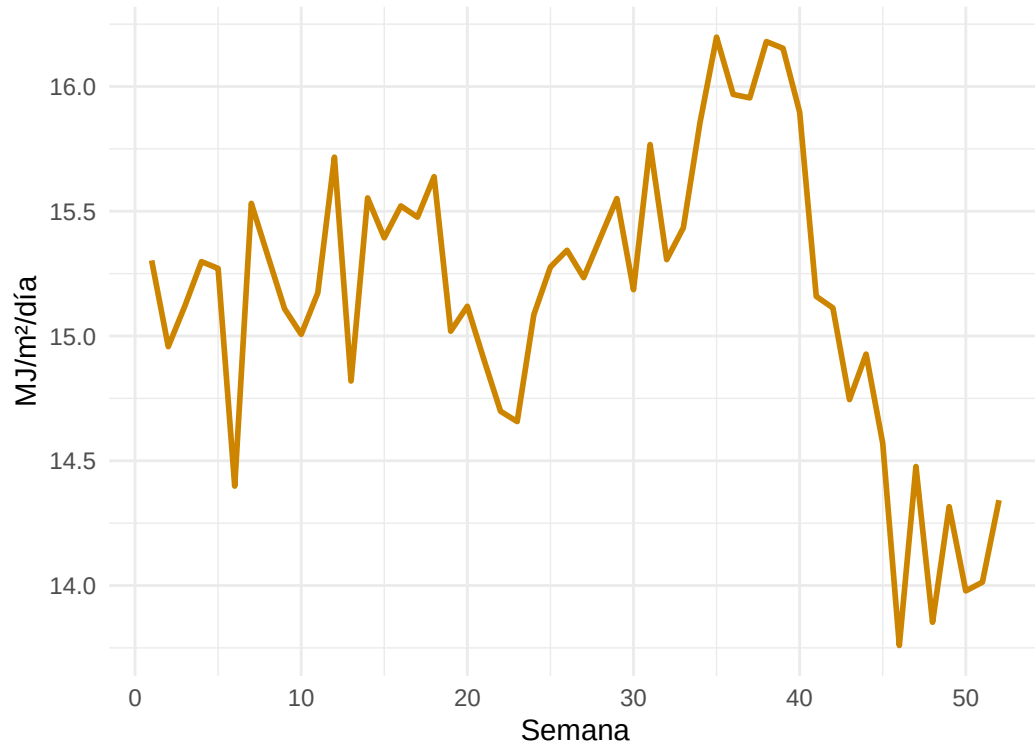
Ciclo climatológico de radiación
