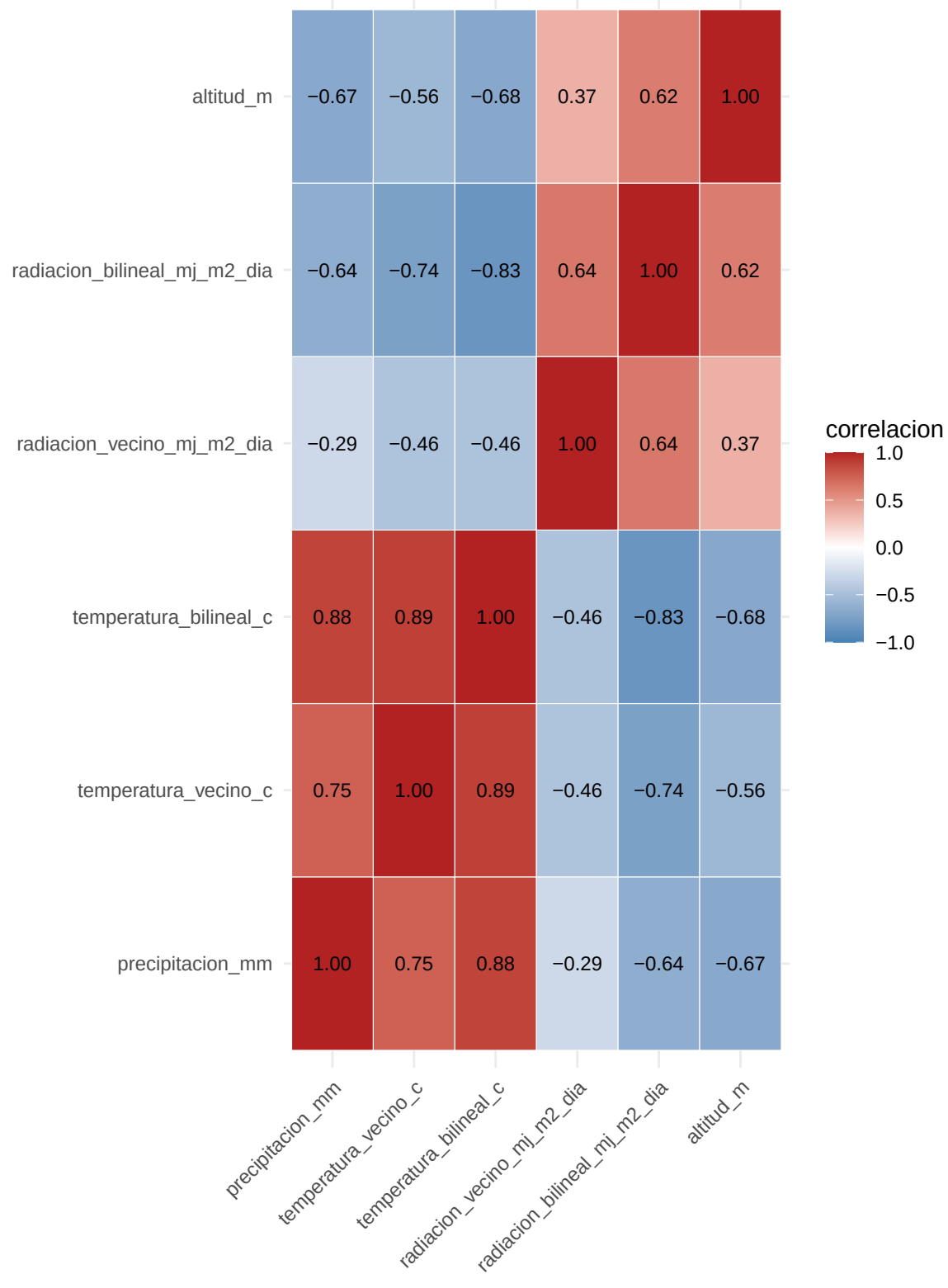
Correlación de promedios espaciales
