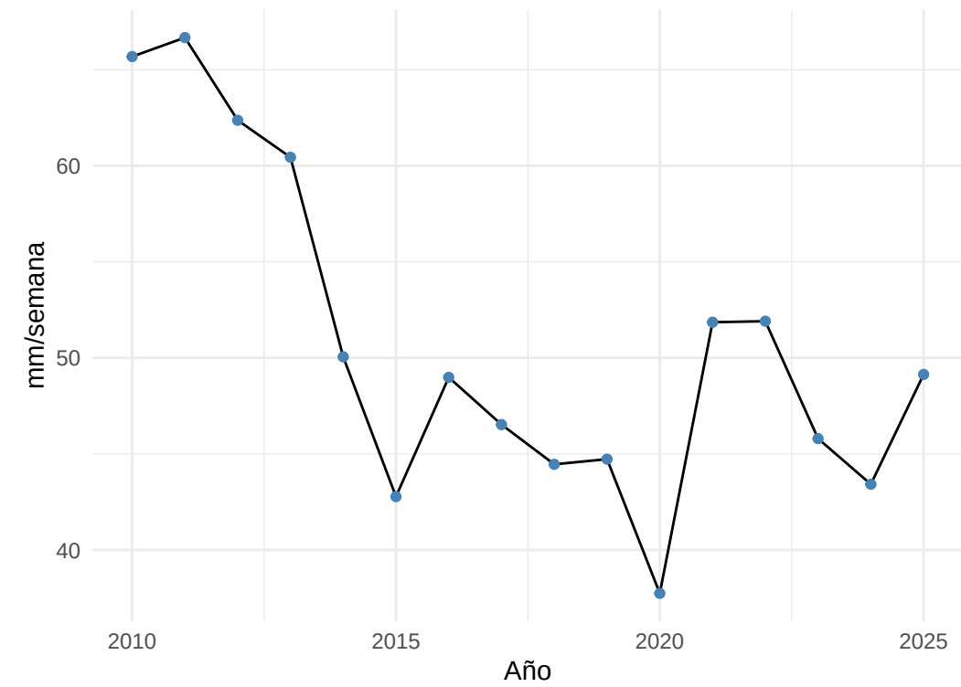
Media anual de precipitación semanal
