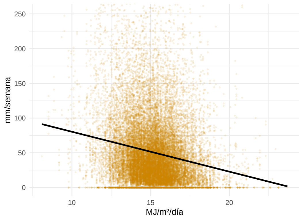
Precipitación vs radiación
