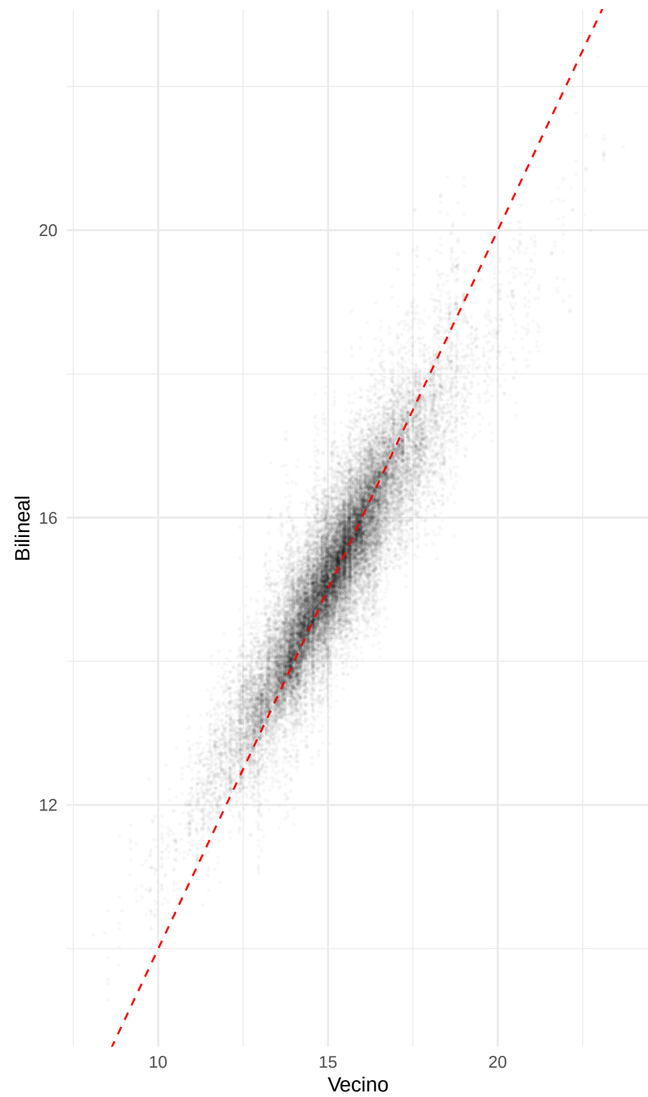
Radiación: vecino vs bilineal
