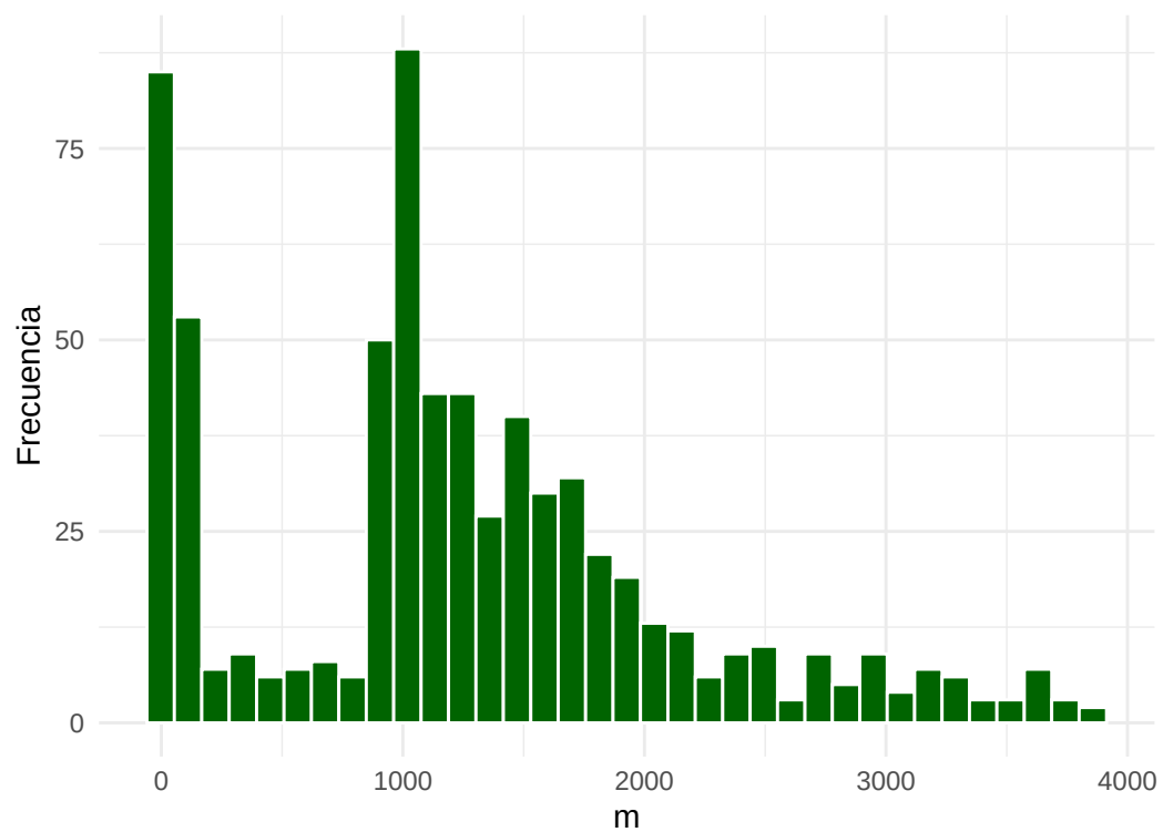
Altitud de las 686 celdas
