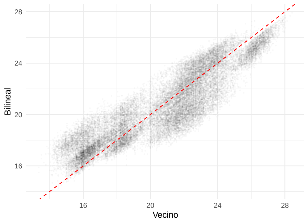
Temperatura: vecino vs bilineal
