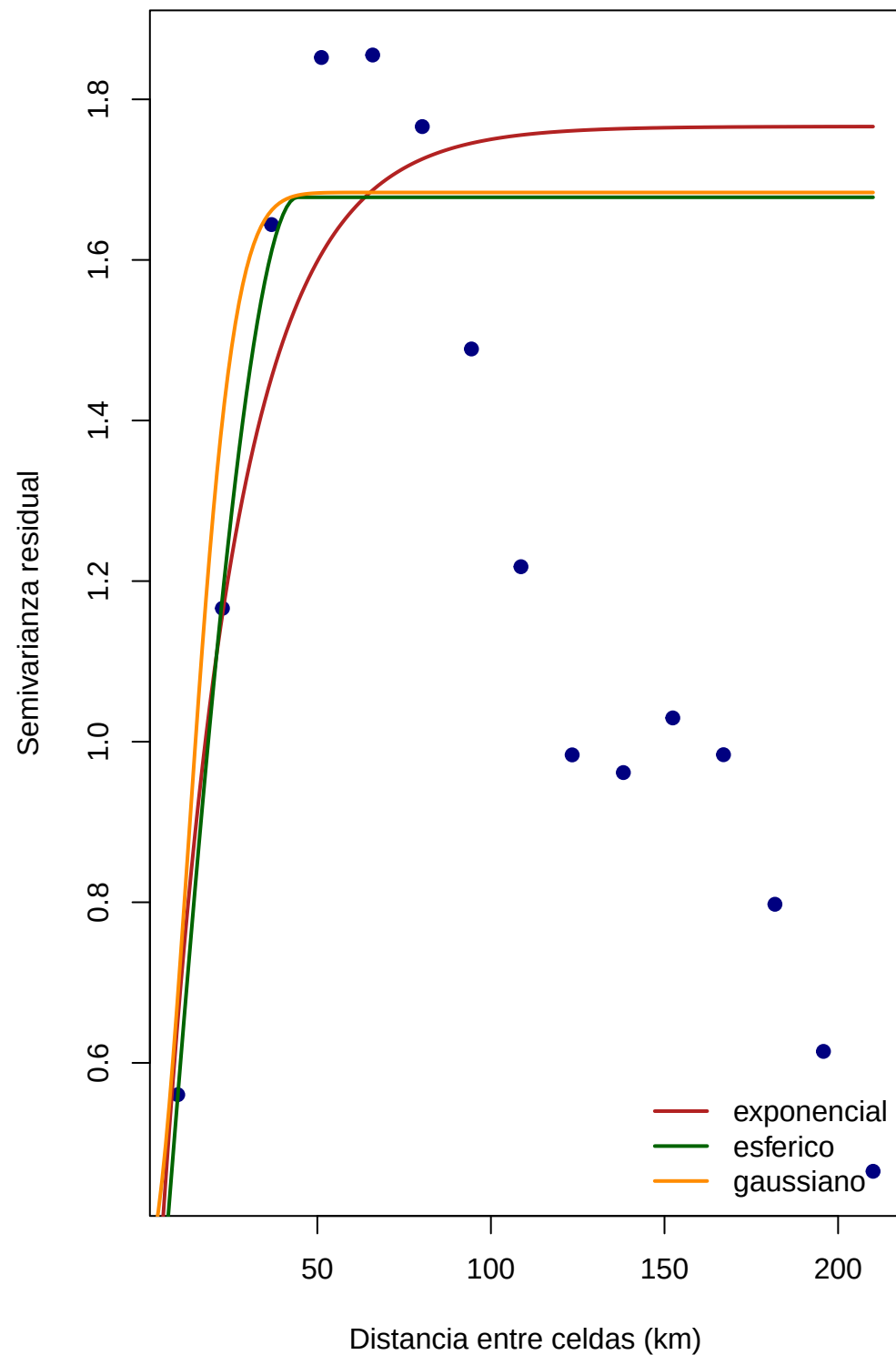
Semivariograma empírico y modelos
