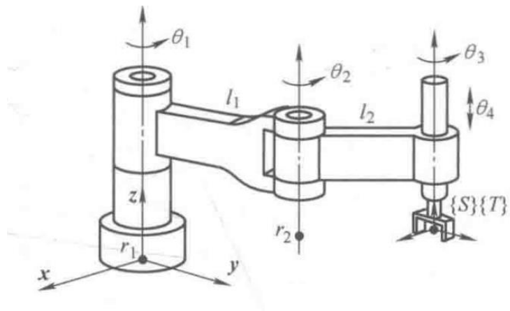
SCARA机器人
