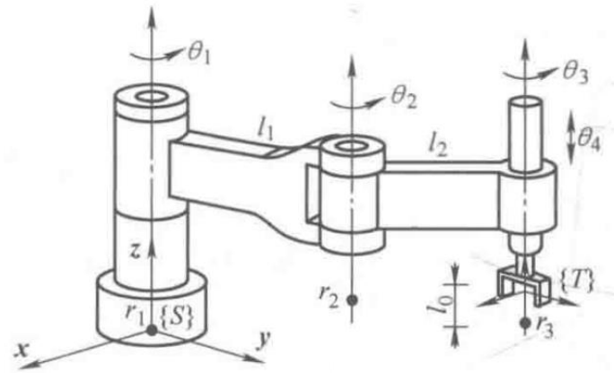
SCARA机器人
