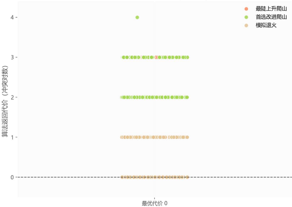
八皇后：算法代价分布 (最优=0)
